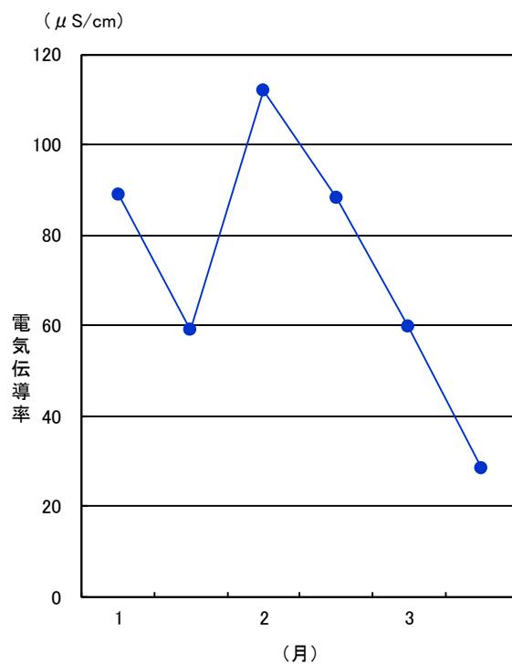
図 1-41 降雪の電気伝導率の推移（令和3年度）
