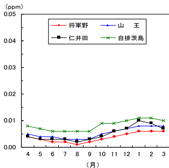
図1-14 二酸化窒素月平均値の変化(令和3年度)
