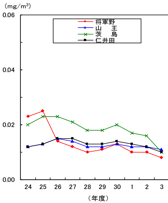
図1-15 浮遊粒子状物質の年平均値の経年変化
