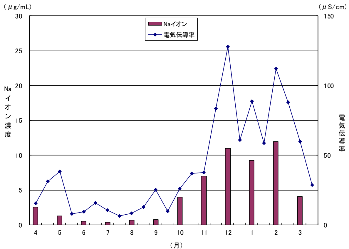
図 1-39 降水の電気伝導率とNaイオン濃度の推移（令和3年度） （4～12月は山王、1～3月は八橋で調査）
