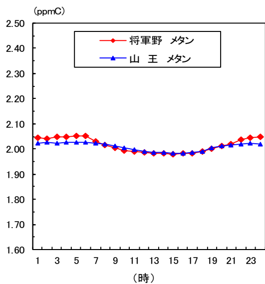
図1－34 メタンの時刻平均値の変化(令和3年度)
