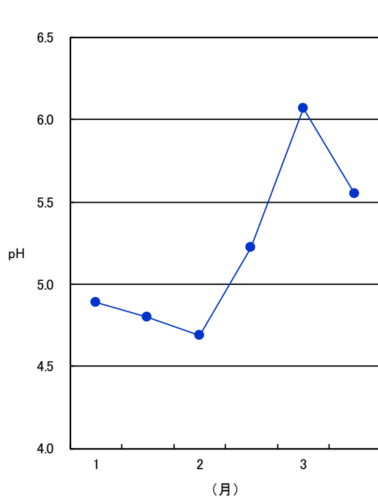
図 1-40 降雪のpHの推移（令和3年度）
