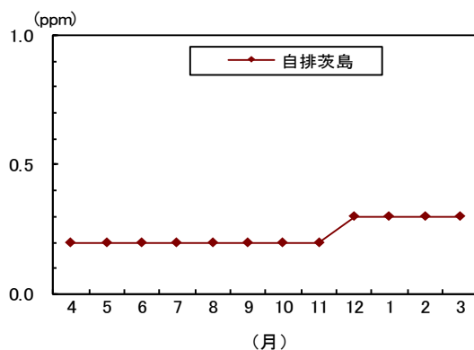
図1-20 一酸化炭素の月平均値の変化
