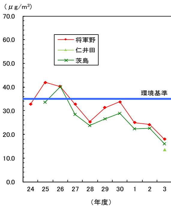
図1-25 微小粒子状物質の日平均値の年間98%値の経年変化
