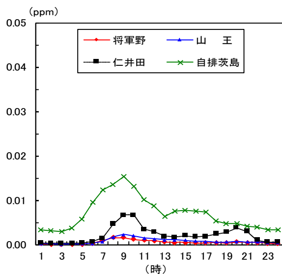
図1-12 一酸化窒素時刻平均値の変化(令和3年度)
