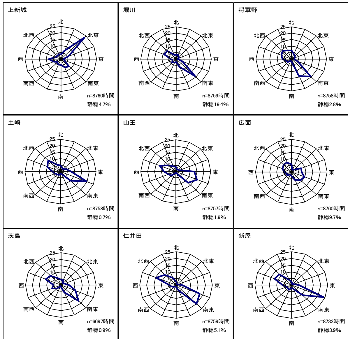
図1－4 風配図 (令和3年度)
