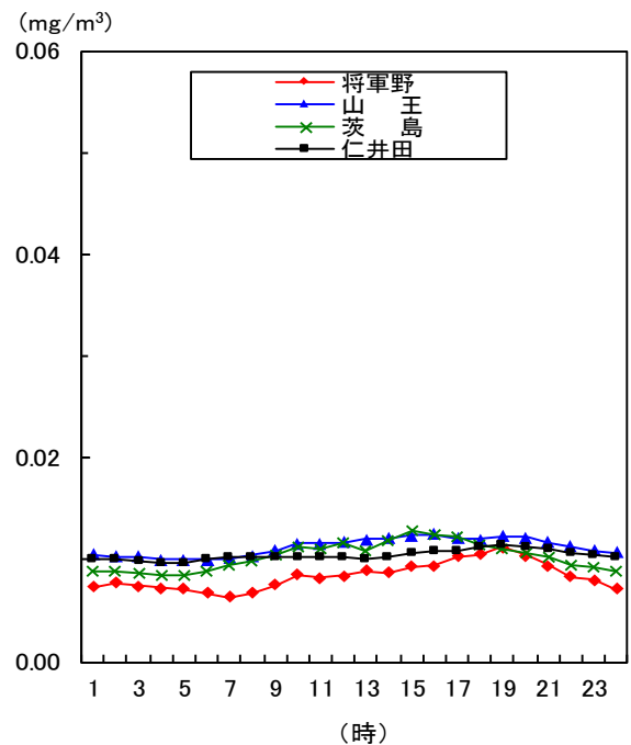
図1-18 浮遊粒子状物質の時刻平均値の変化 (令和3年度)
