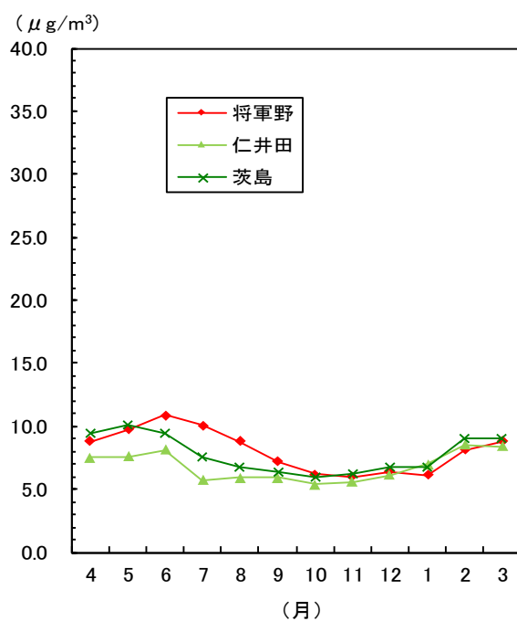
図1-26 微小粒子状物質の月平均値の変化 (令和3年度)
