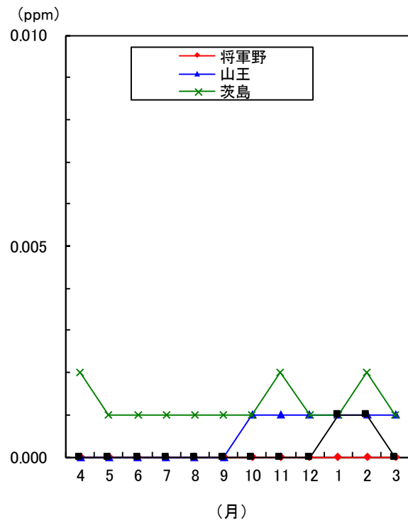
図1-8 二酸化硫黄月平均値の変化(令和3年度)
