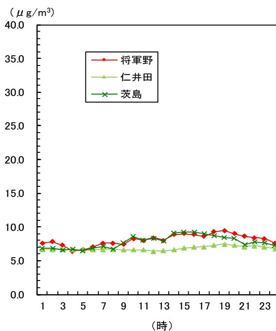
図1-27 微小粒子状物質の時刻平均値の変化 (令和3年度)
