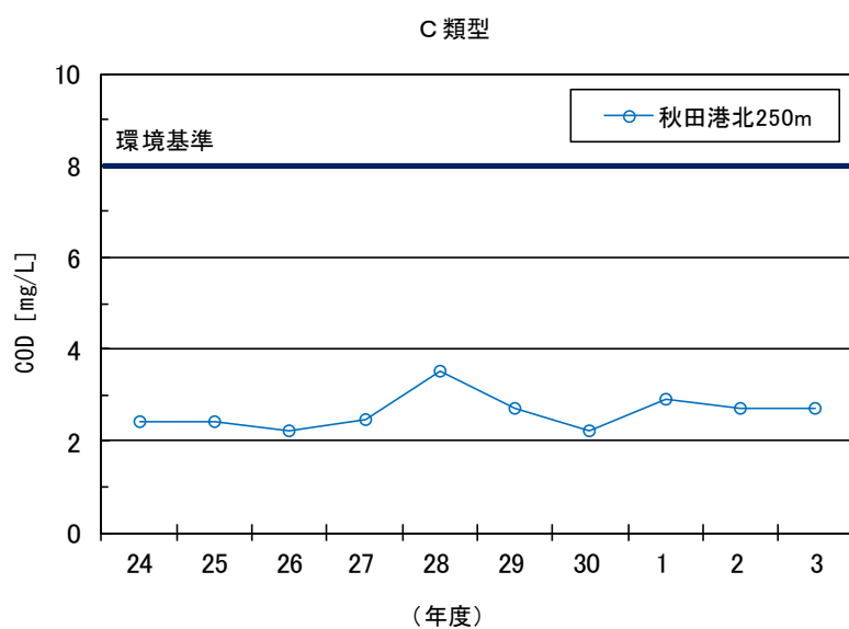
図 2 - 3 海域のCOD75%値の経年変化
