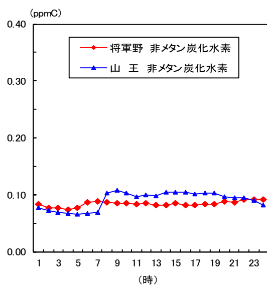
図1－33 非メタン炭化水素の時刻平均値の変化 (令和3年度)
