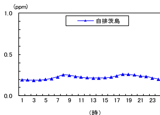
図1-21 一酸化炭素の時刻平均値の変化
