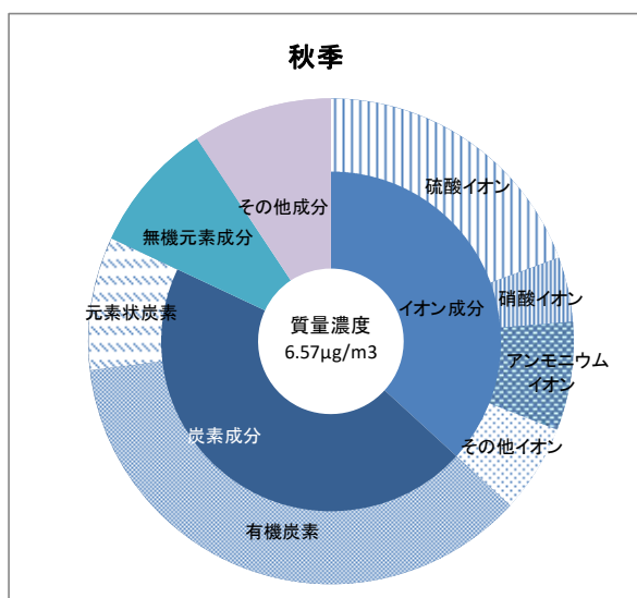
図1-30 PM2.5成分分析結果(秋季)(令和3年度)
