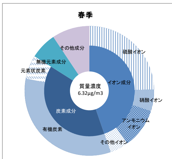
図1-28 PM2.5成分分析結果(春季)(令和3年度)
