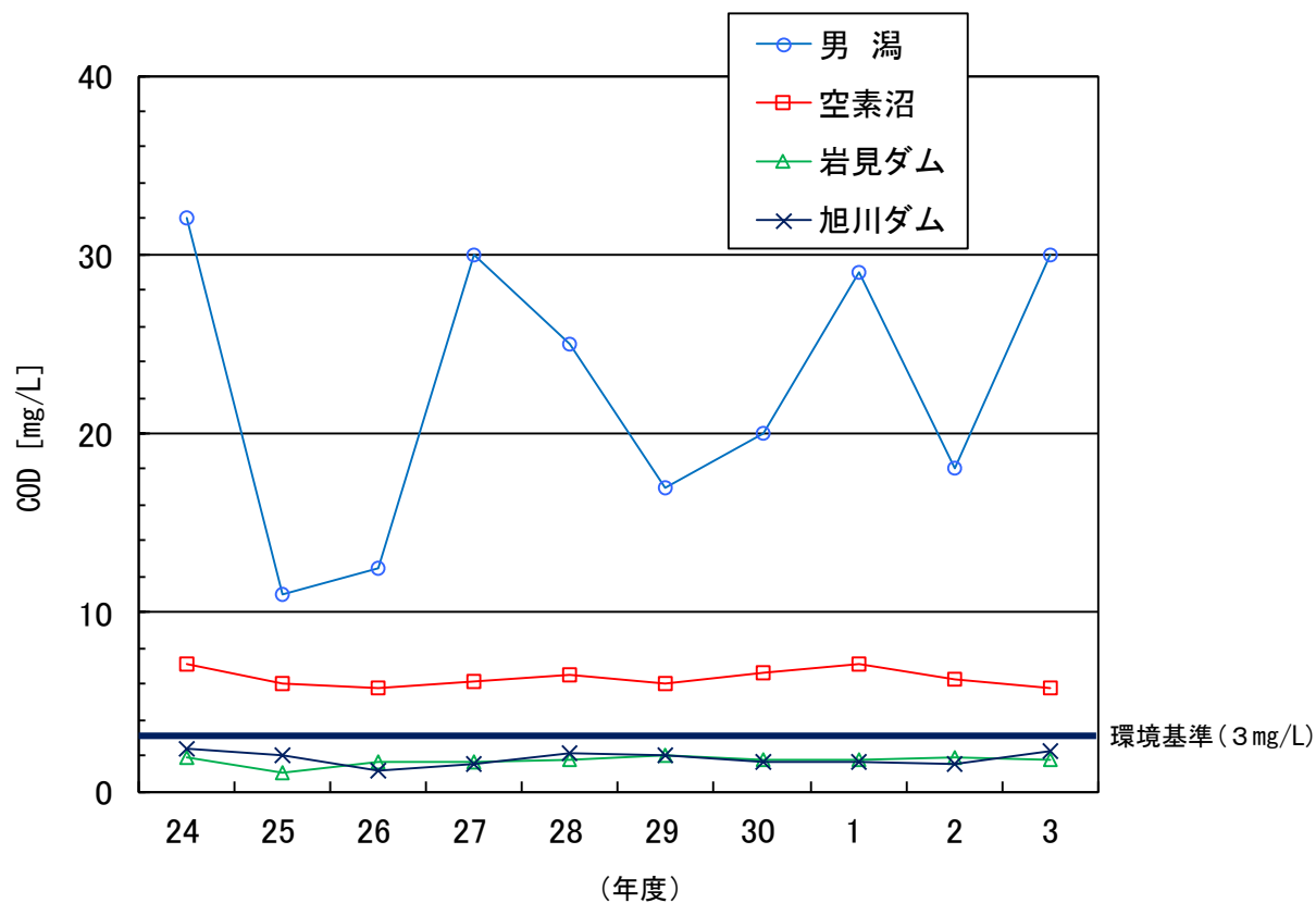
図 2-4 湖沼のCOD75%値の経年変化
