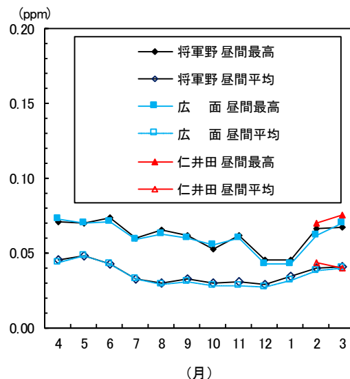
図1-23 光化学オキシダントの月平均値の変化（令和3年度）
