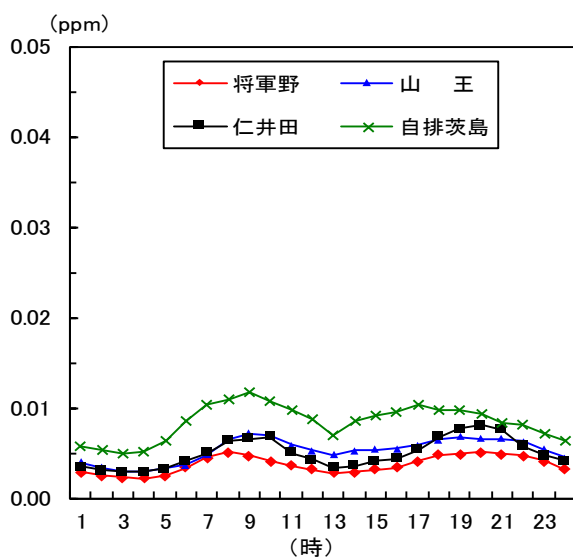
図1-13 二酸化窒素時刻平均値の変化(令和3年度)
