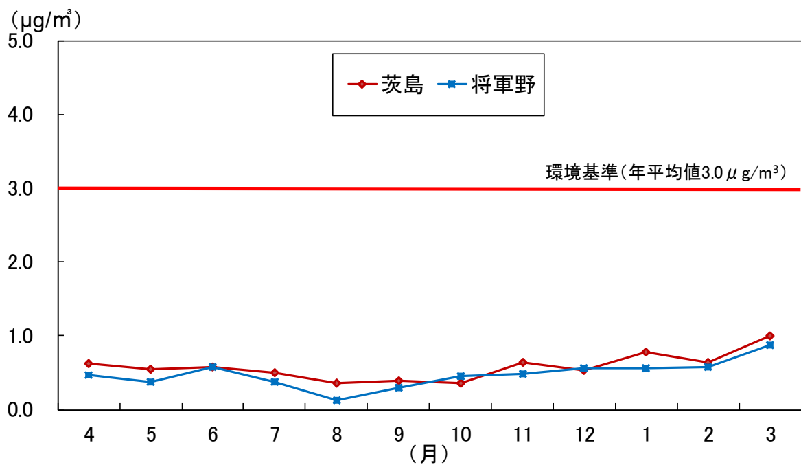
図 1-36 ベンゼンの測定結果（令和 3 年度）
