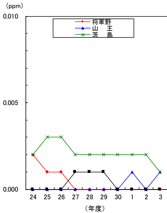
図1-6 二酸化硫黄年平均値の経年変化
