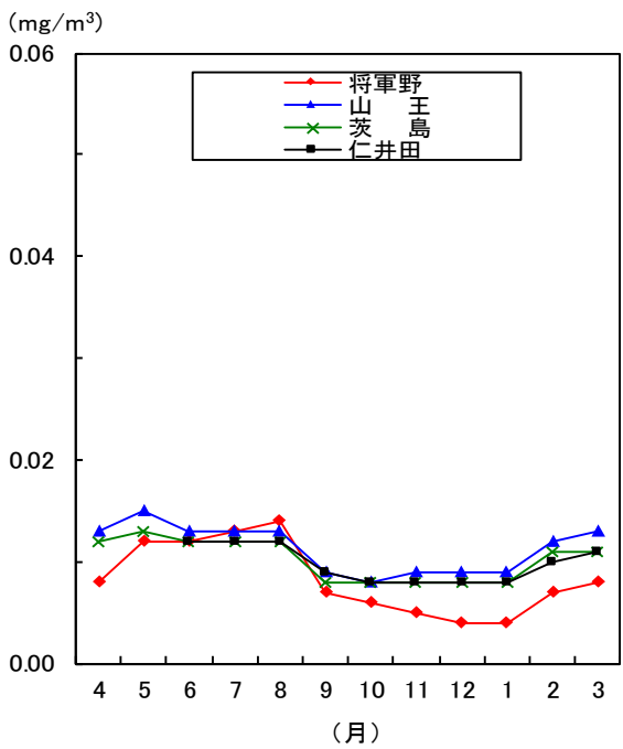
図1-17 浮遊粒子状物質の月平均値の変化 (令和3年度)
