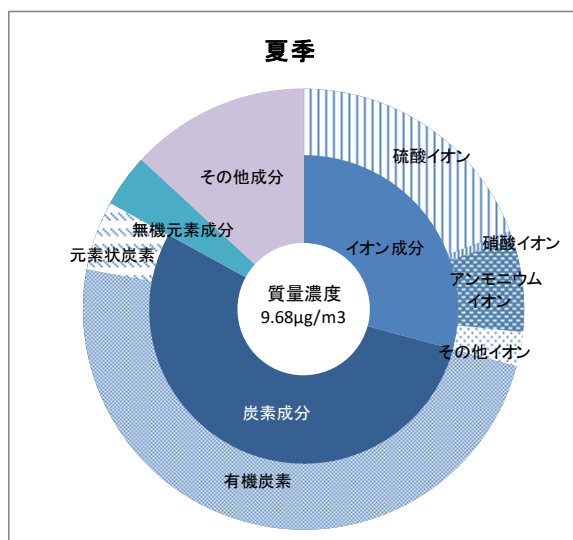
図1-29 PM2.5成分分析結果(夏季)(令和3年度)
