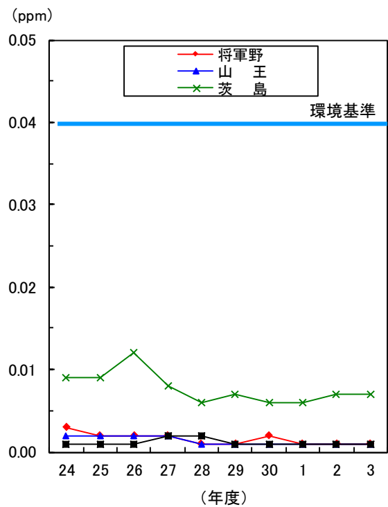
図1-7 二酸化硫黄日平均値の2%除外値の経年変化
