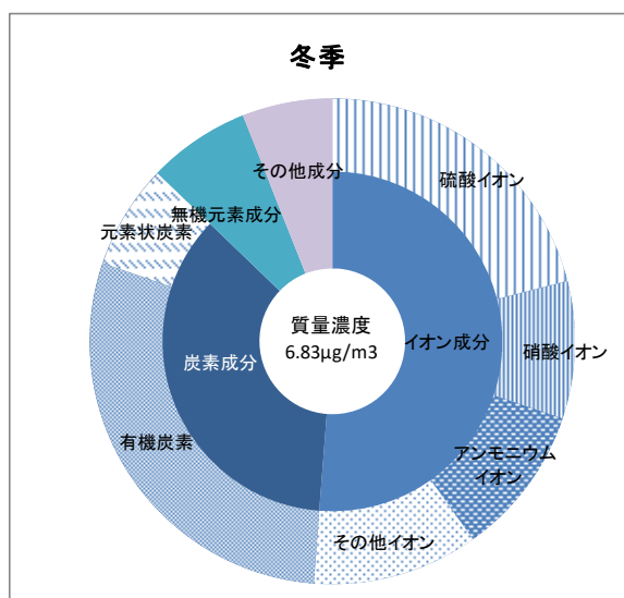
図1-31 PM2.5成分分析結果(冬季)(令和3年度)
