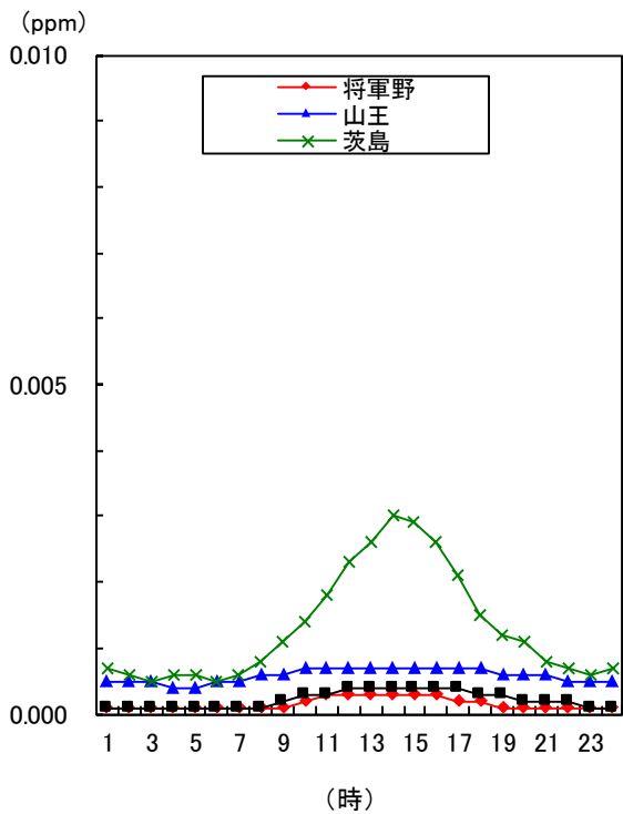
図1-9 二酸化硫黄時刻平均値の変化(令和3年度)
