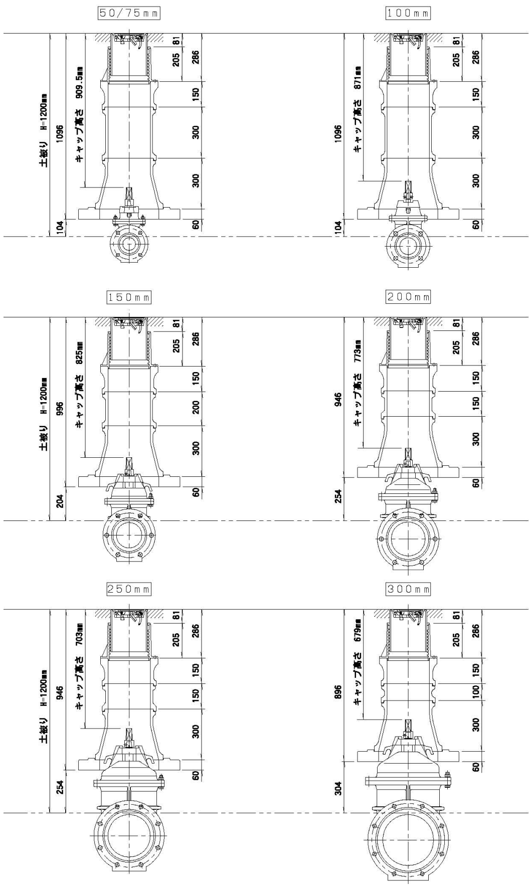
仕切弁きょう浅層埋設対応標準図 (H=1200)
