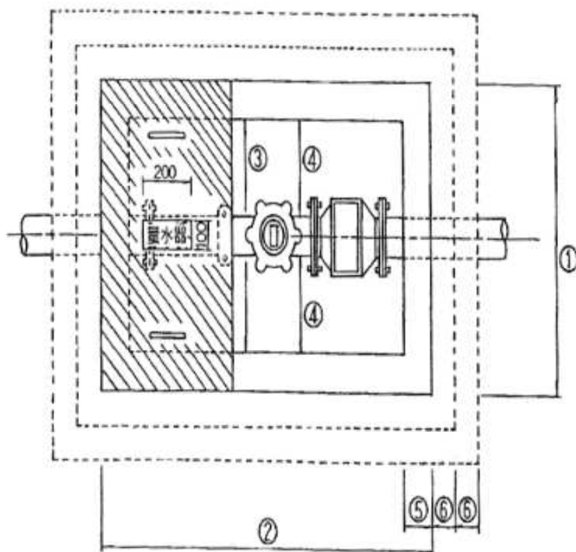
平面图
