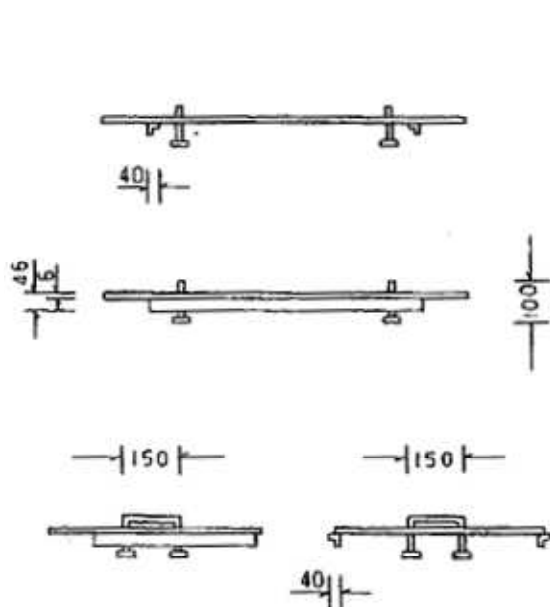
断面図（大蓋）
