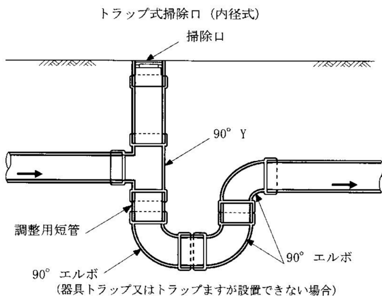
図4-43 トラップ付掃除口の例
