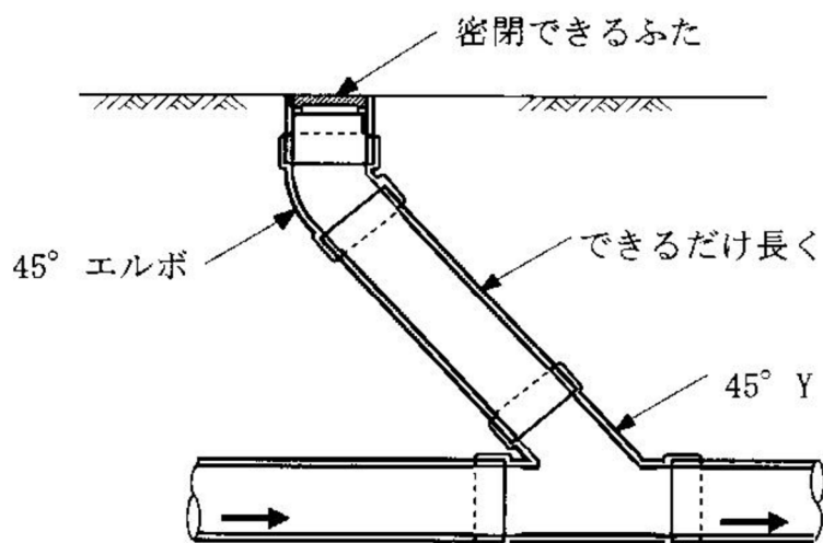
図4-42 掃除口の例（ますが設置できない場合）
