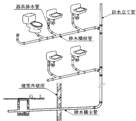
図 4－１ 排水管の種類
