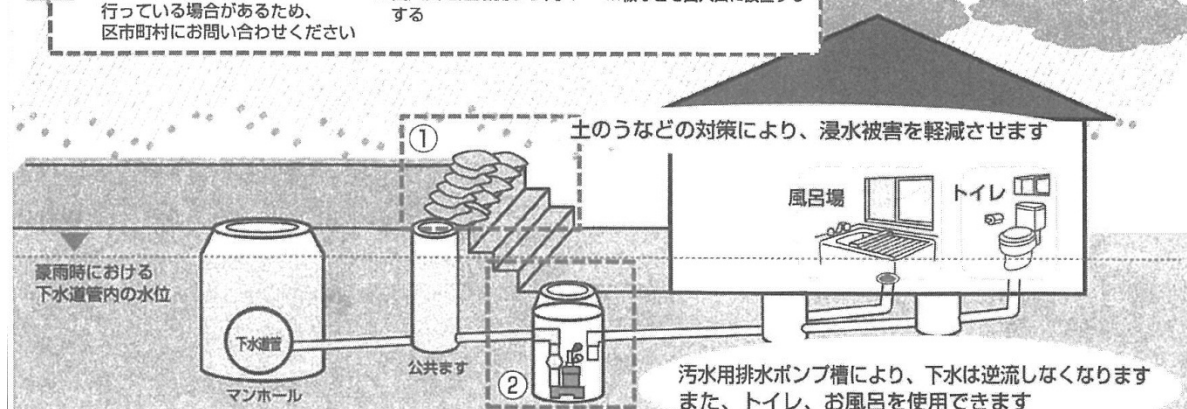
図 8 - 2 半地下家屋浸水対策事例
