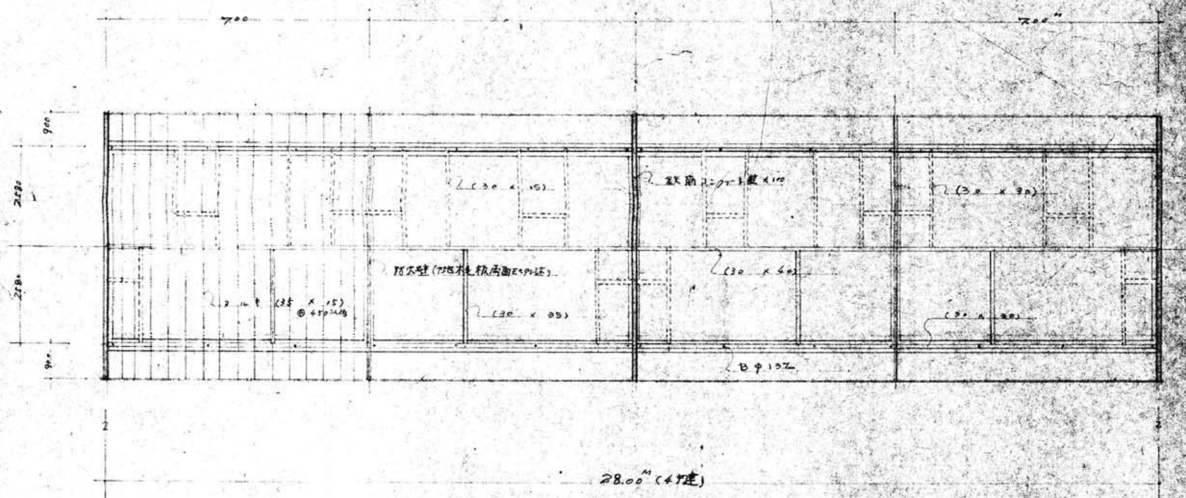
小屋伏 (取組伏図) S.1:100
