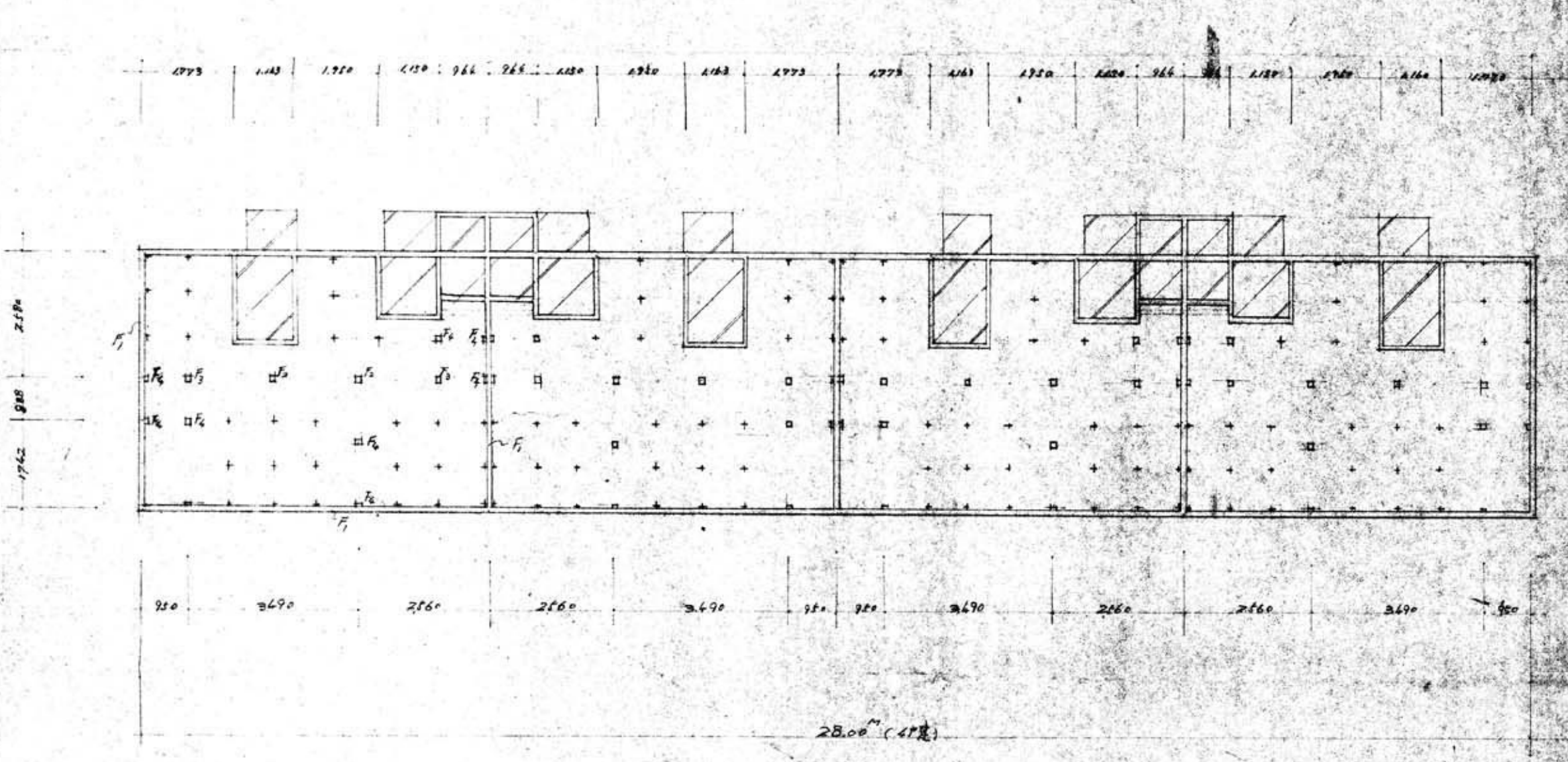
基礎伏図 S.1:100
