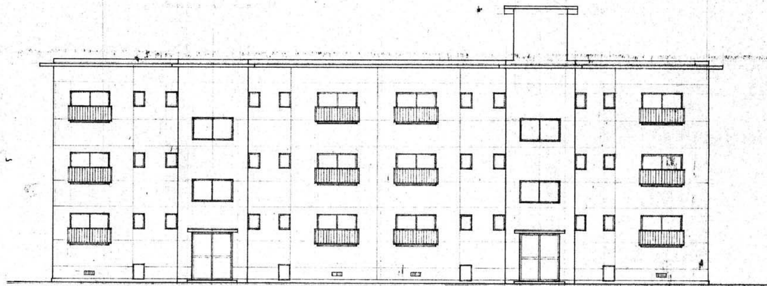
北立面图
