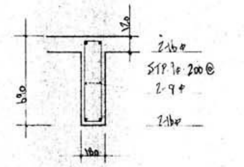
(3階梁伏図) RB
