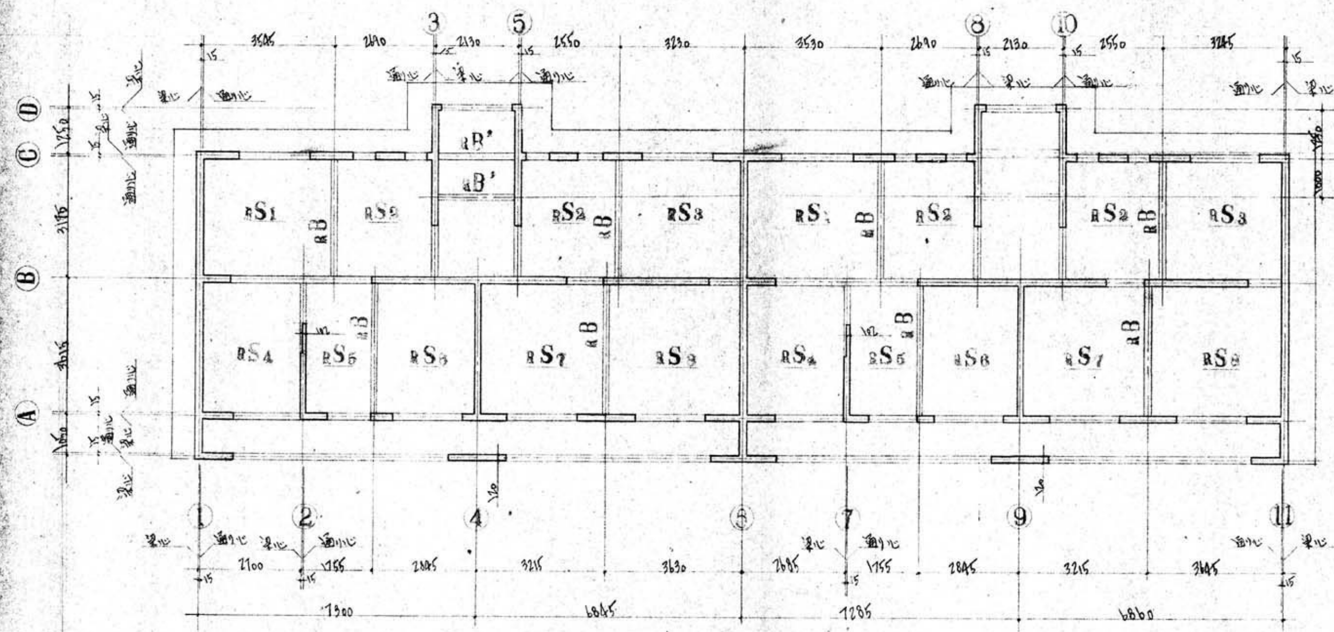
R階梁伏図
