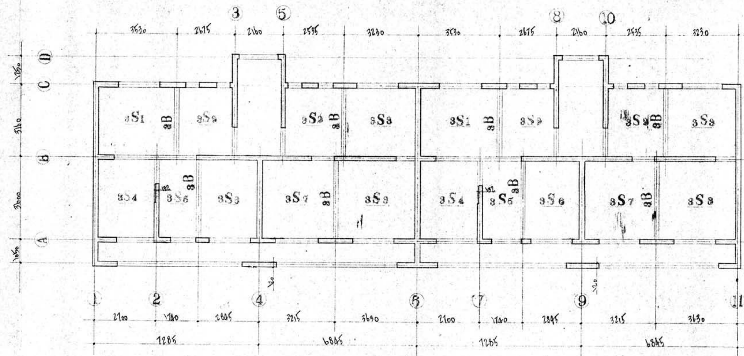
3階梁伏図
