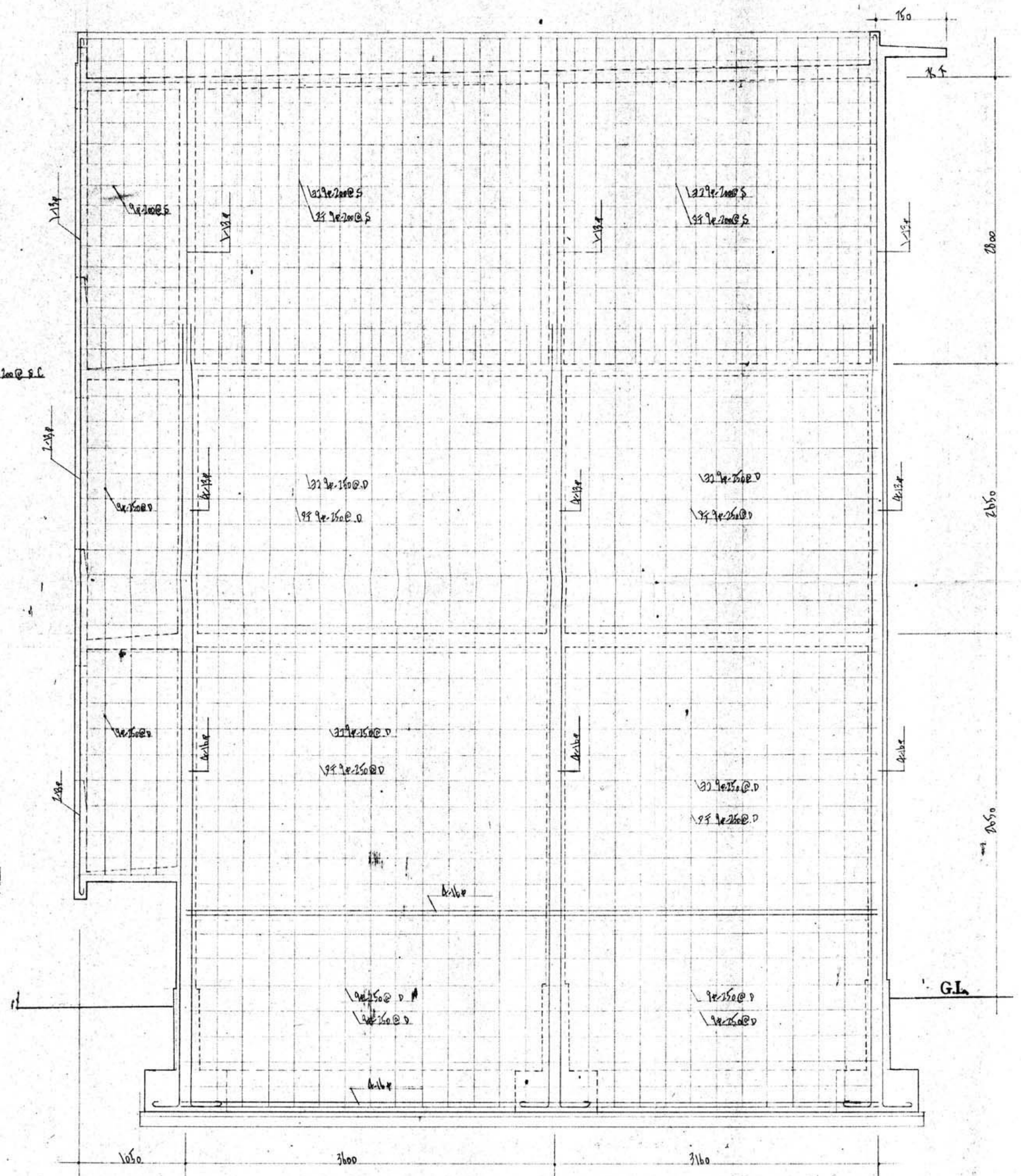
1.1.2 配筋詳細図 1/30
