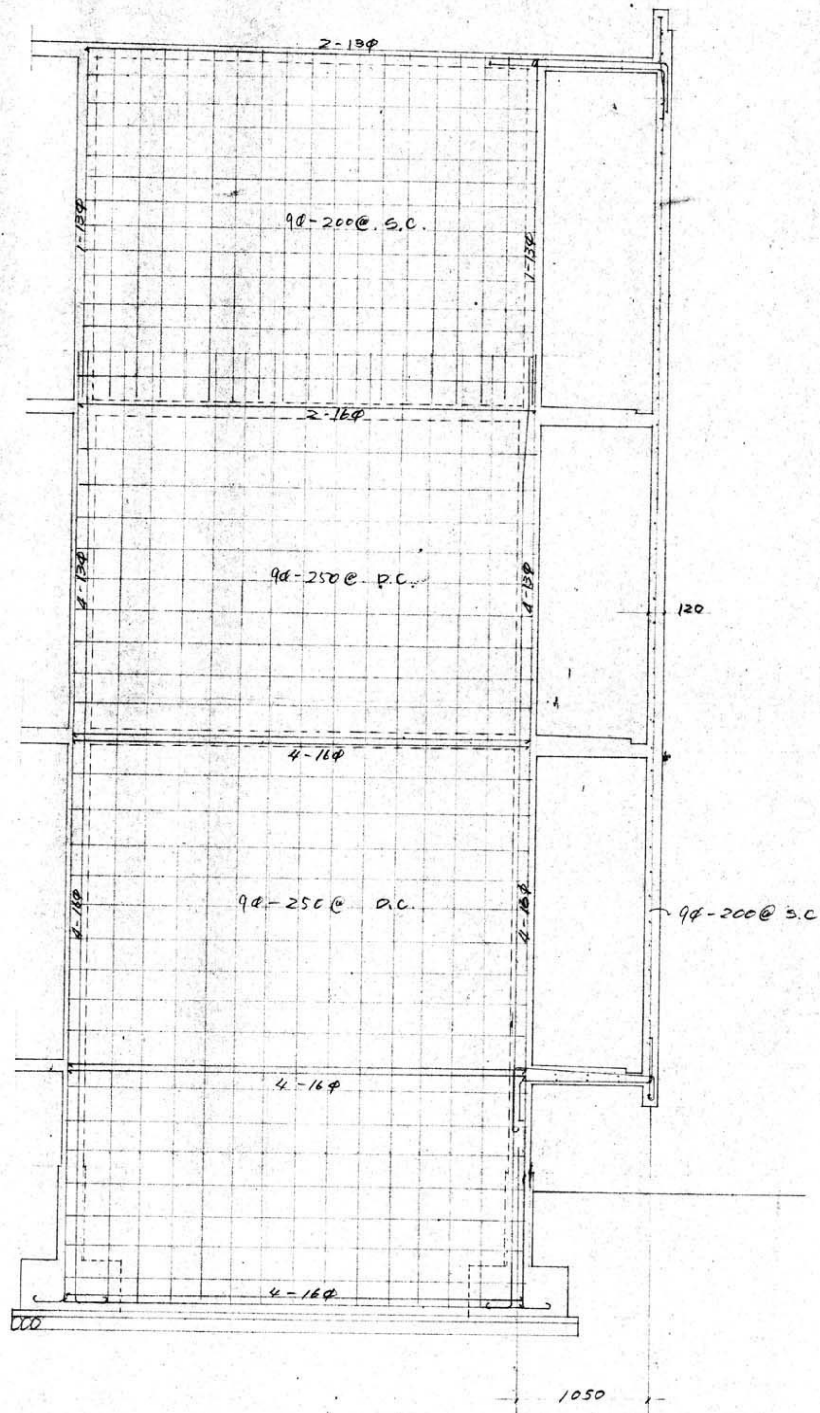
4. 9. 通り配筋詳細図 1/30
