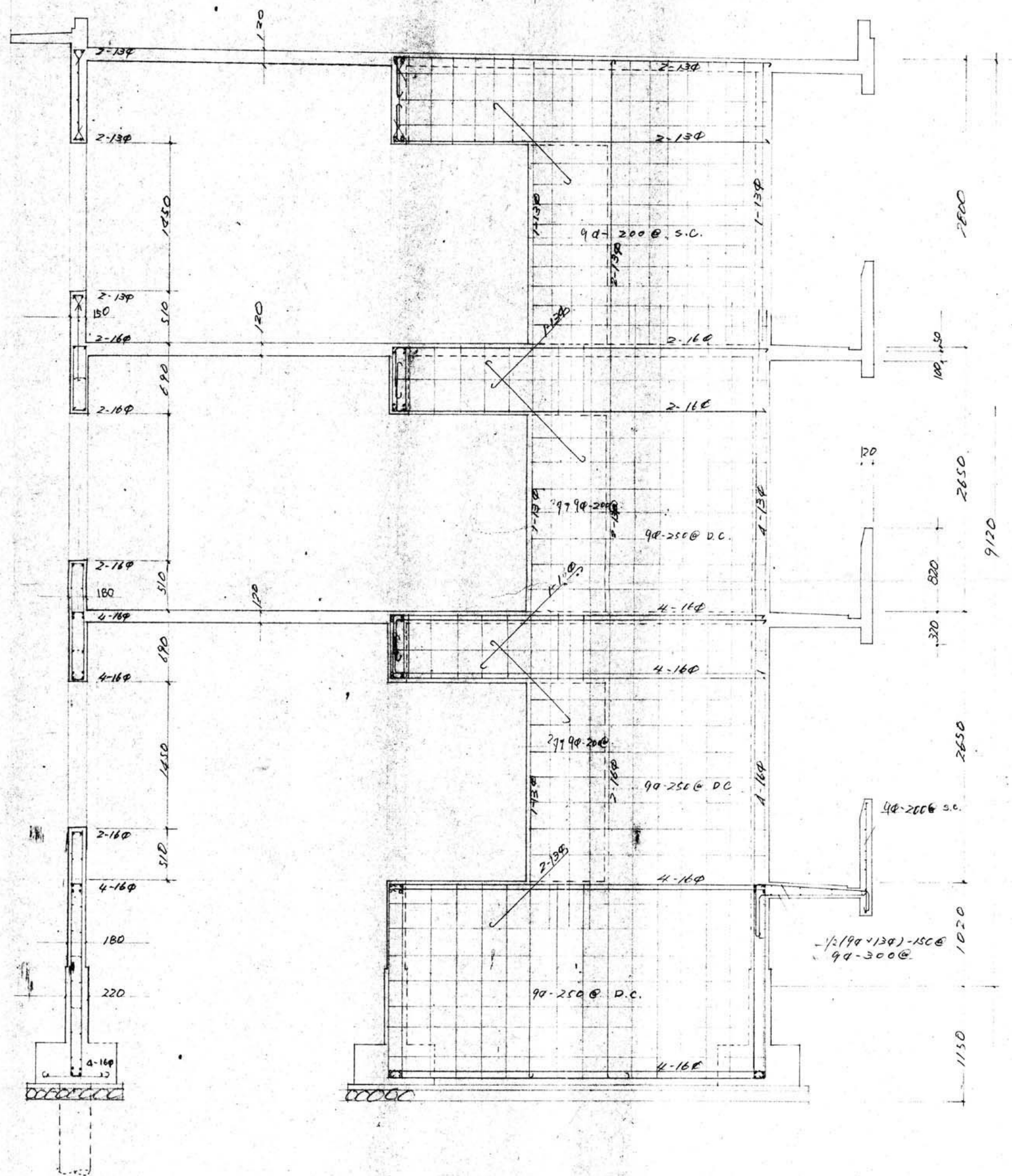
2. 7. 通り配筋詳細図 1/30
