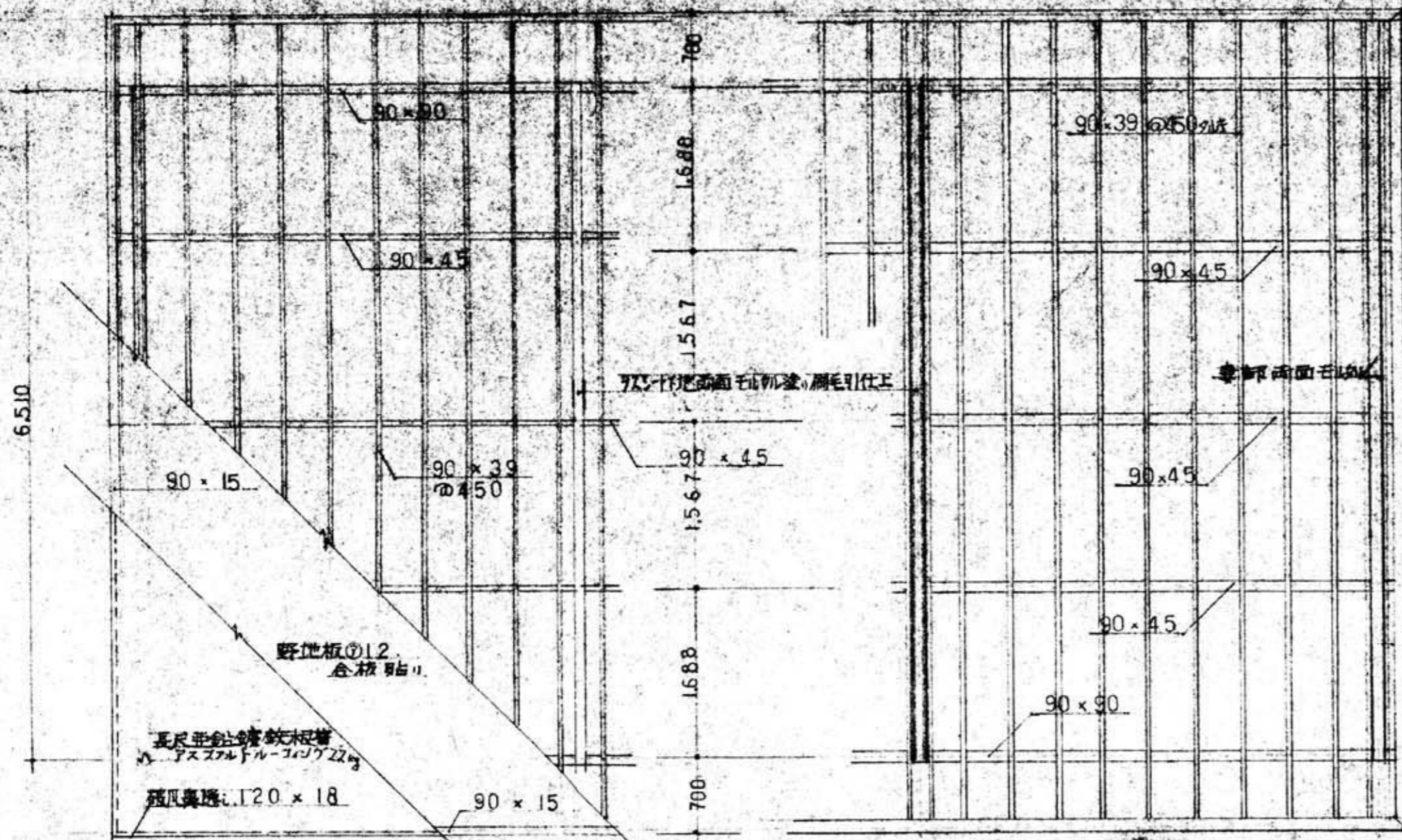
2種小屋伏図
