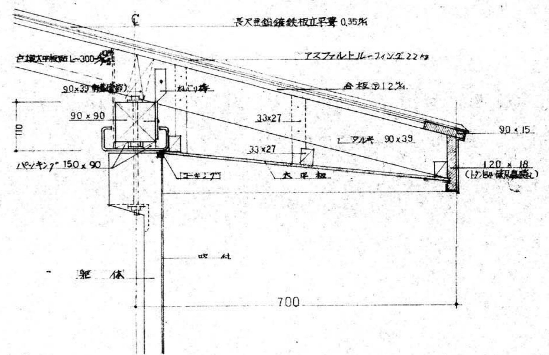
軒折まわり
