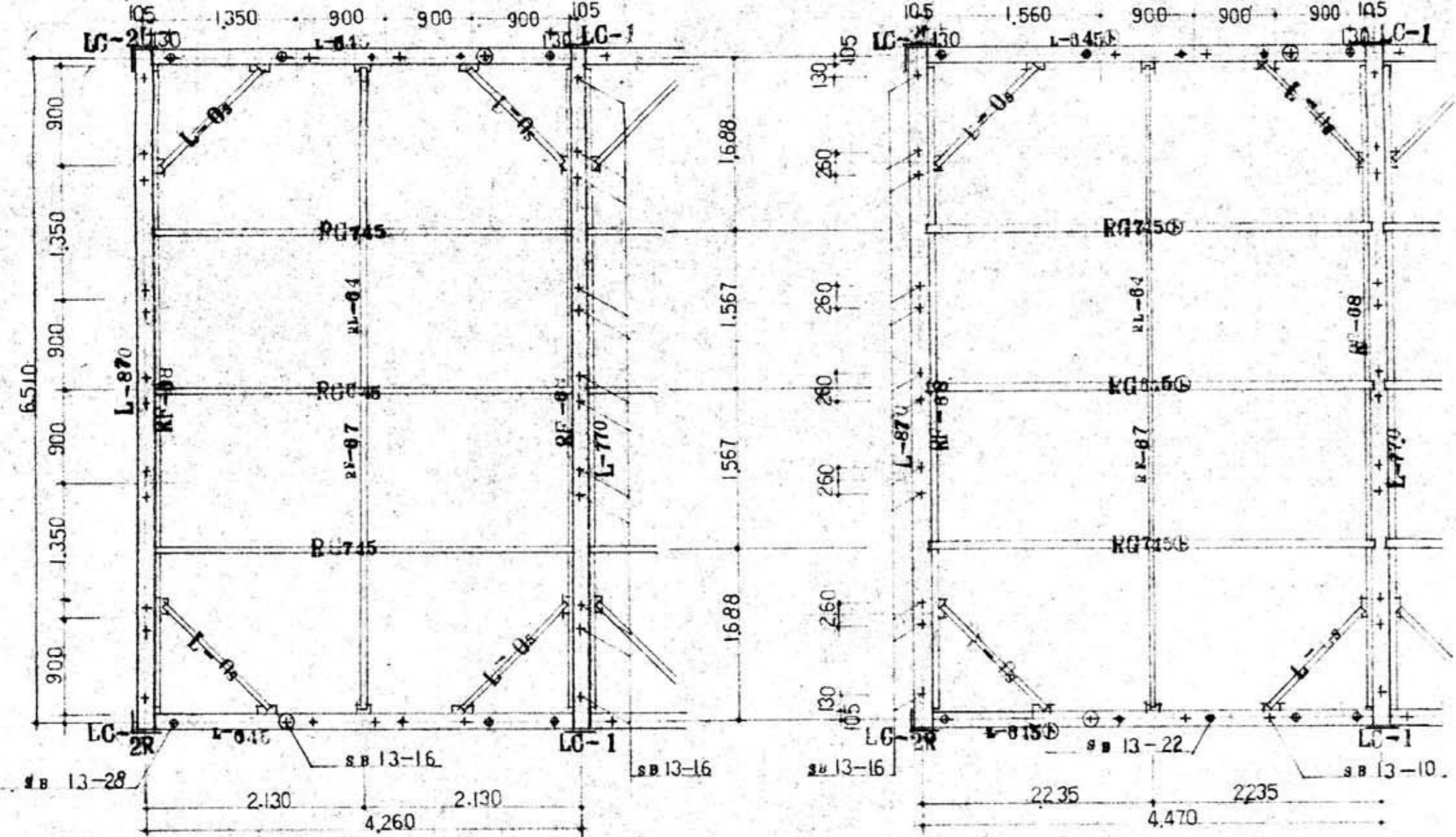
2種小屋梁伏図
