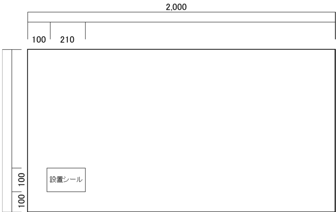
標識盤面図(裏)
