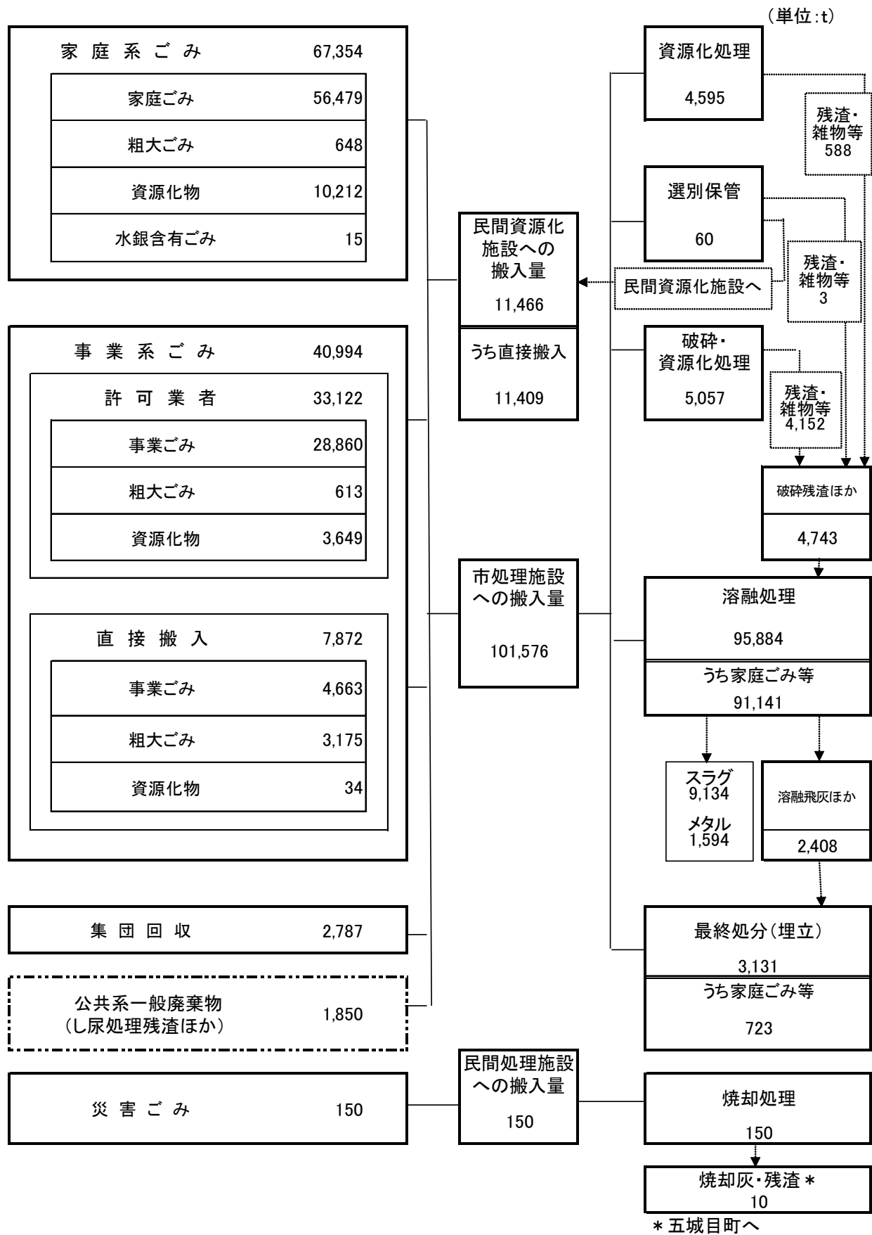
(参考) ゴミ処理計画フロー図
