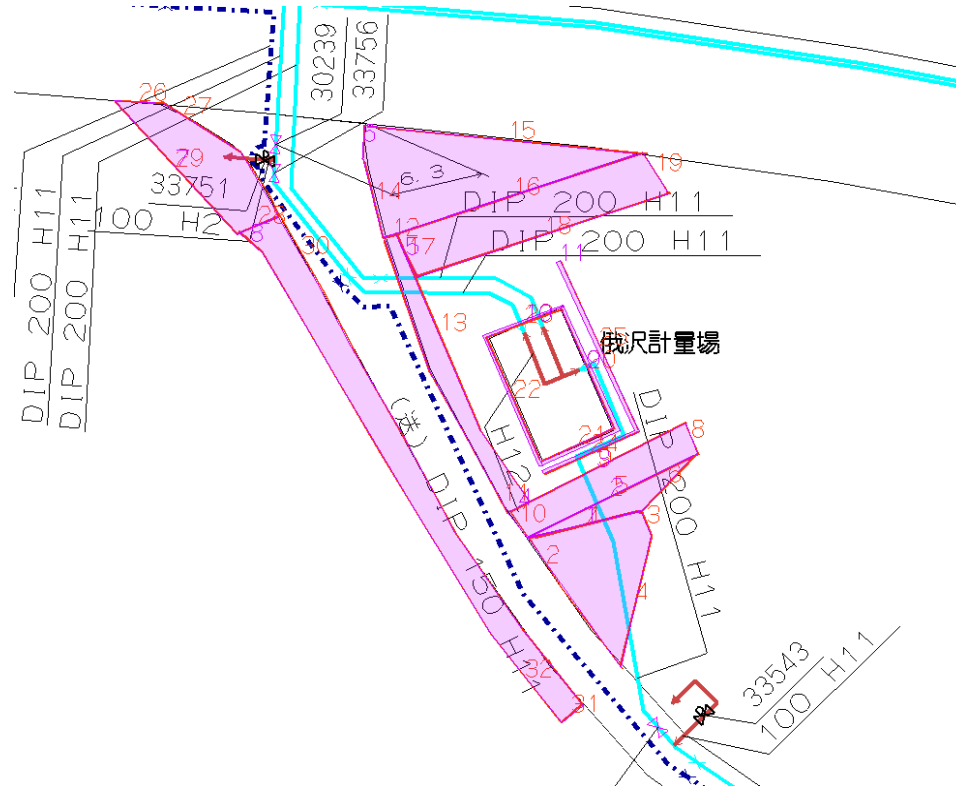
平面図
