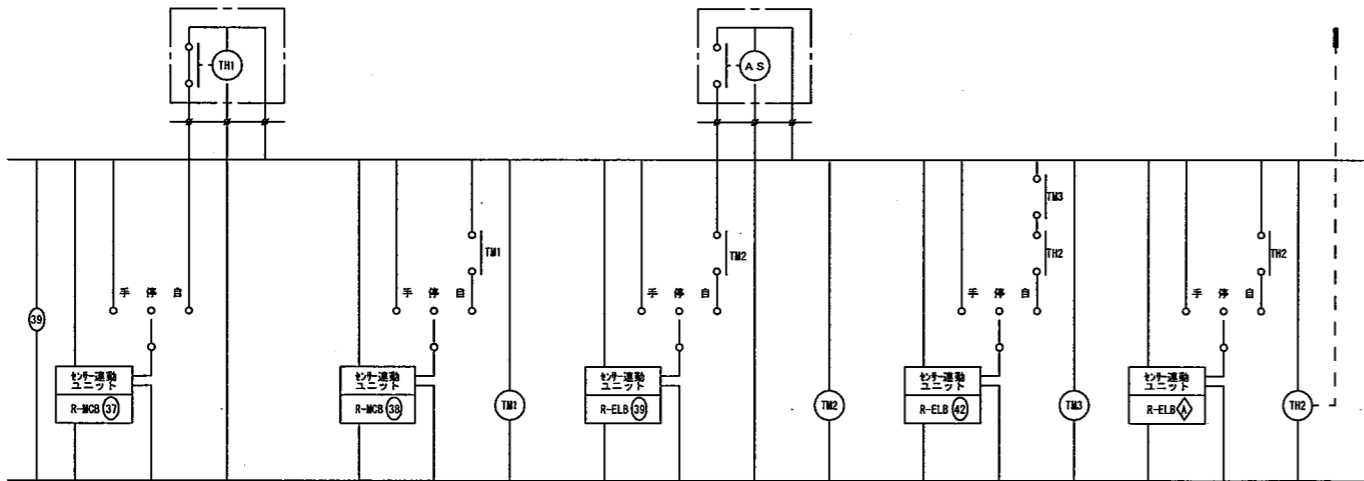
電灯動力分電盤 (S-1LP-1) 結線図
