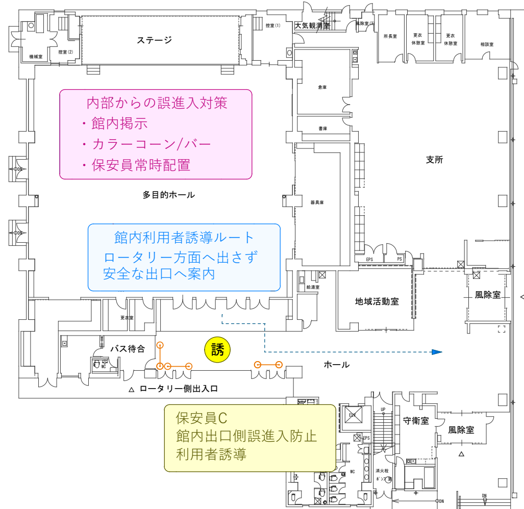
1階平面図
