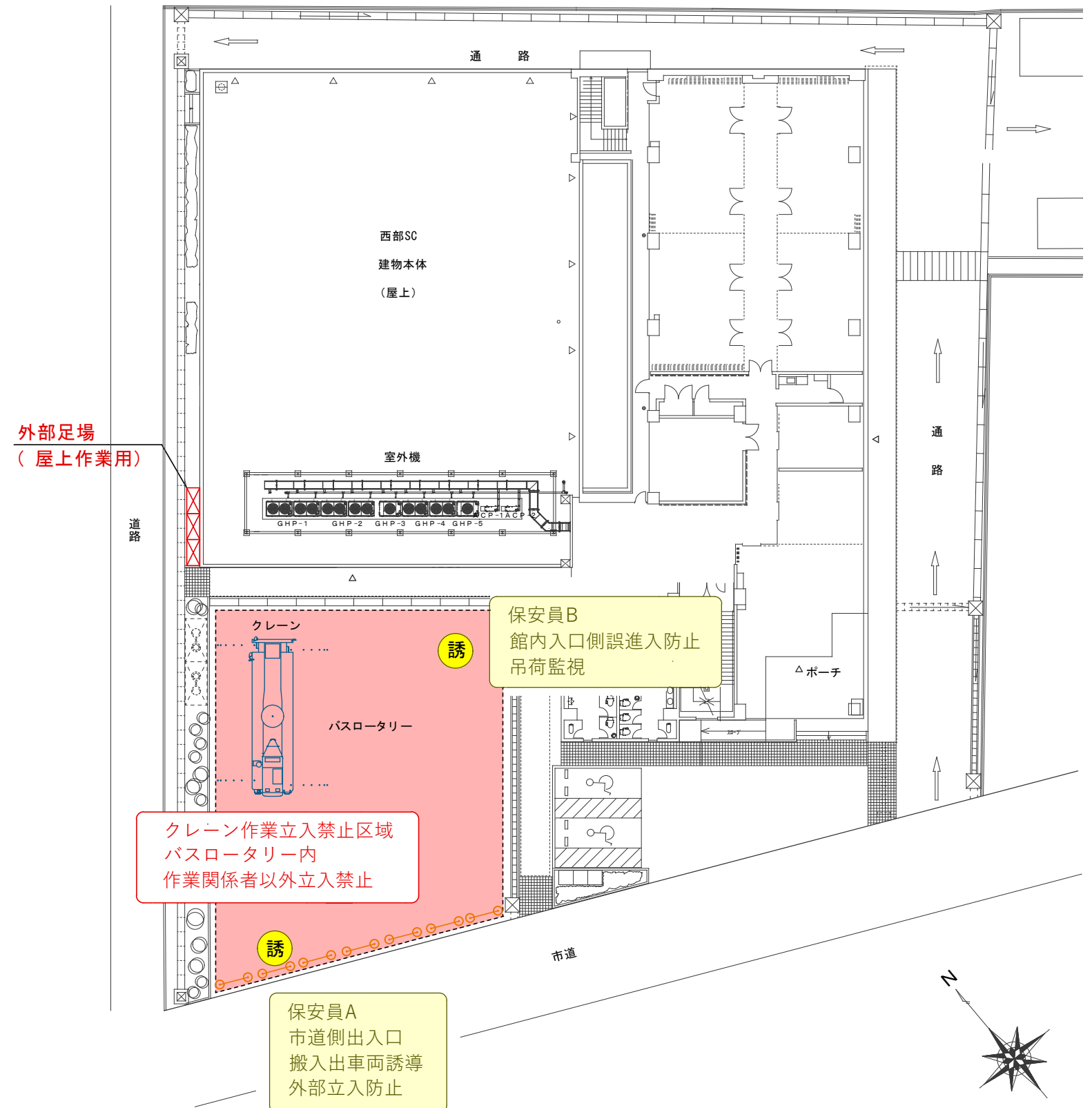
外部クレーン配置図
