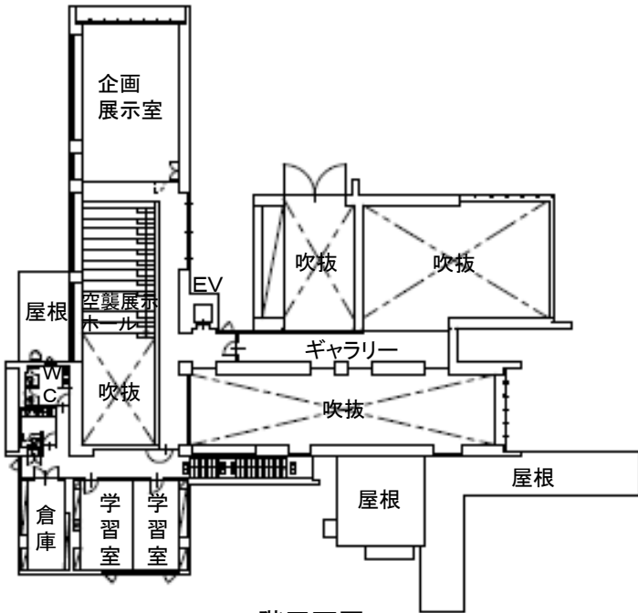
2階平面図
