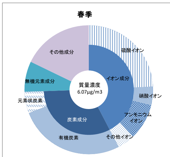
図1-28 PM2.5成分分析結果(春季)(令和2年度)
