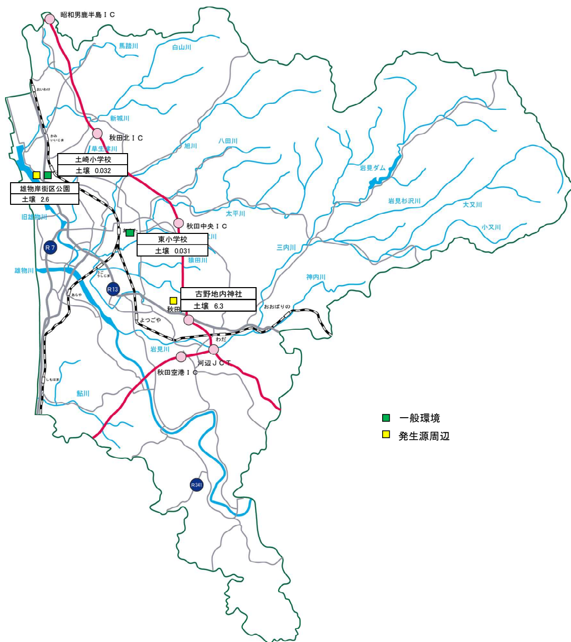
図 5－3 環境中のダイオキシン類測定地点図（土壌関係）
