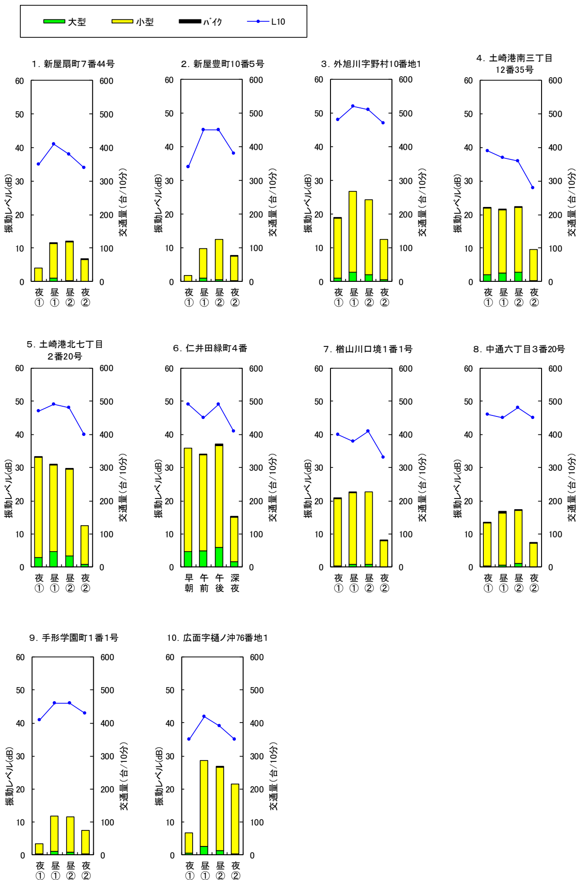
図3-4 道路交通振動と交通量の時間区分別変化（令和2年度）
