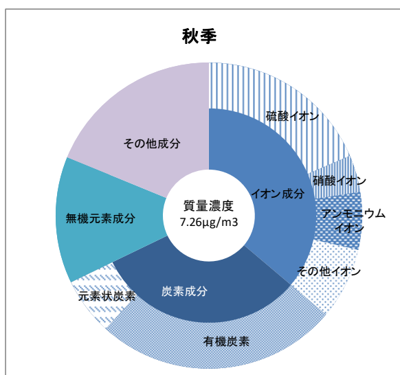
図1-30 PM2.5成分分析結果(秋季)(令和2年度)
