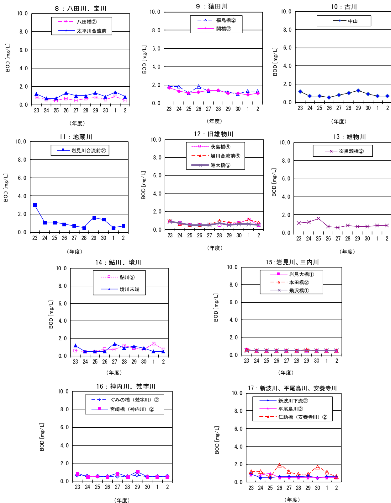
図 2-3 BOD 75% 値の過去 10 年間の比較 (2)
