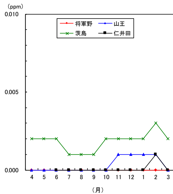
図1-8 二酸化硫黄月平均値の変化(令和2年度)
