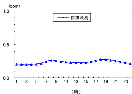
図1-21 一酸化炭素の時刻平均値の変化 （令和2年度）
