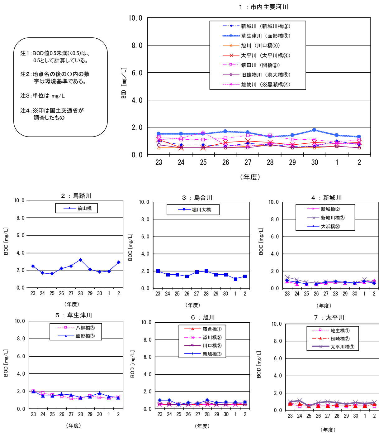
図 2 - 3 BOD 75%値の過去 10 年間の比較(1)
