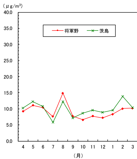
図1-26 微小粒子状物質の月平均値の変化 (令和2年度)
