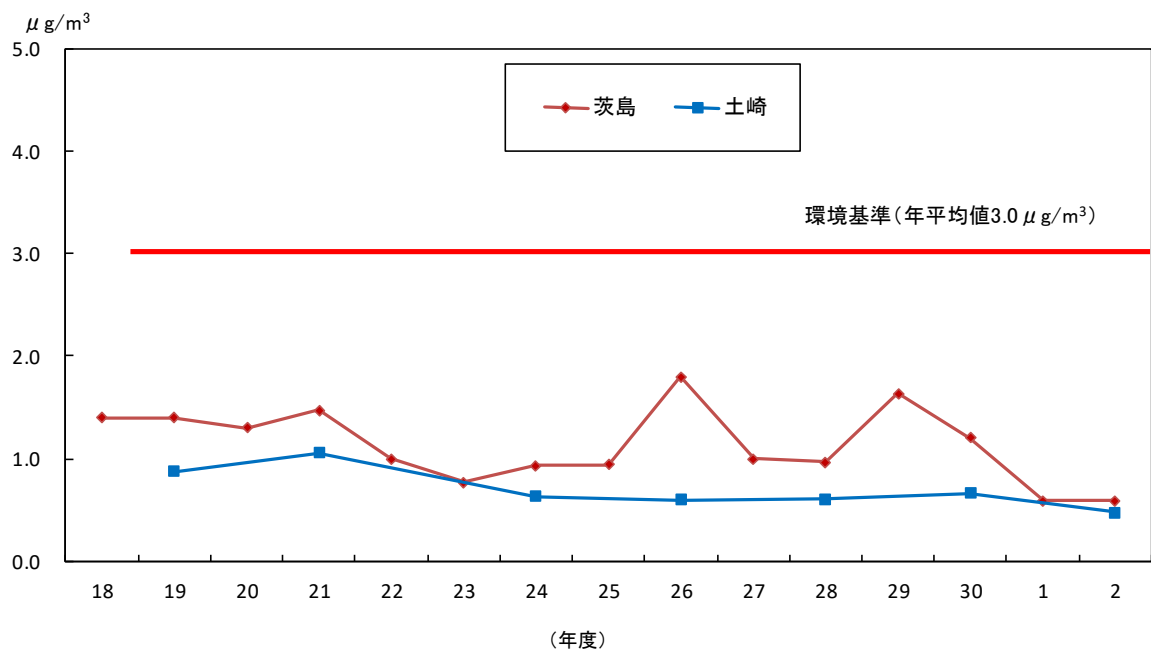
図1-35 ベンゼンの年平均値の経年変化
