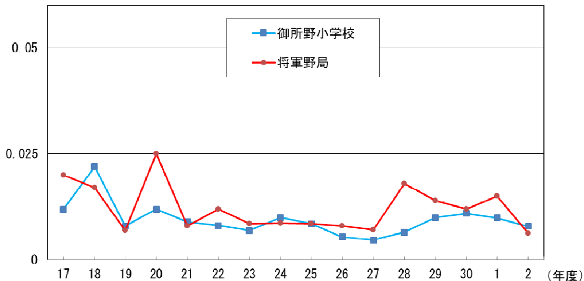
図5－1 大気中のダイオキシン類濃度の推移
