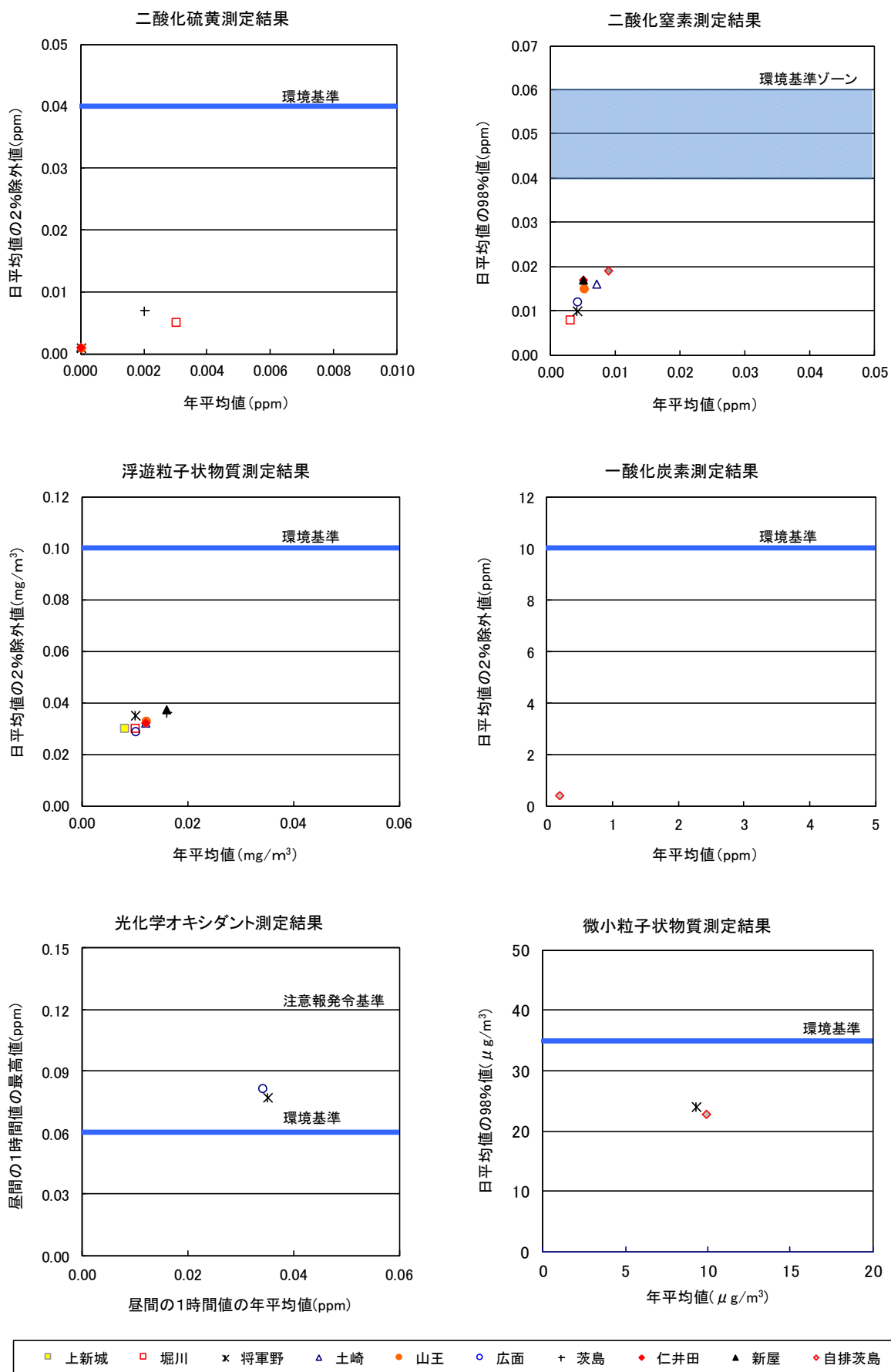
図 1 - 3 大気環境基準の達成状況 (令和2年度)
