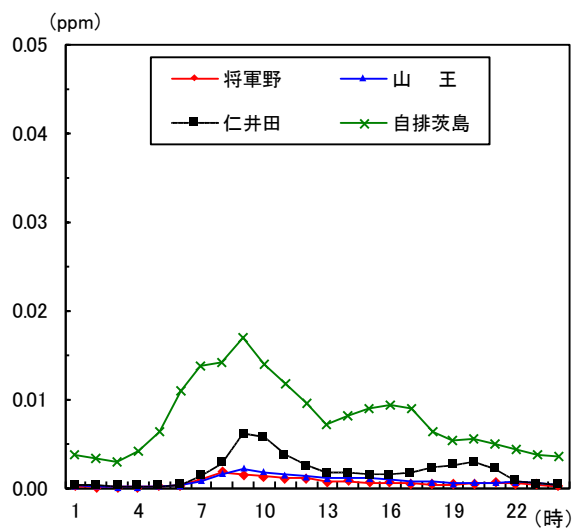
図1-12 一酸化窒素時刻平均値の変化(令和2年度)
