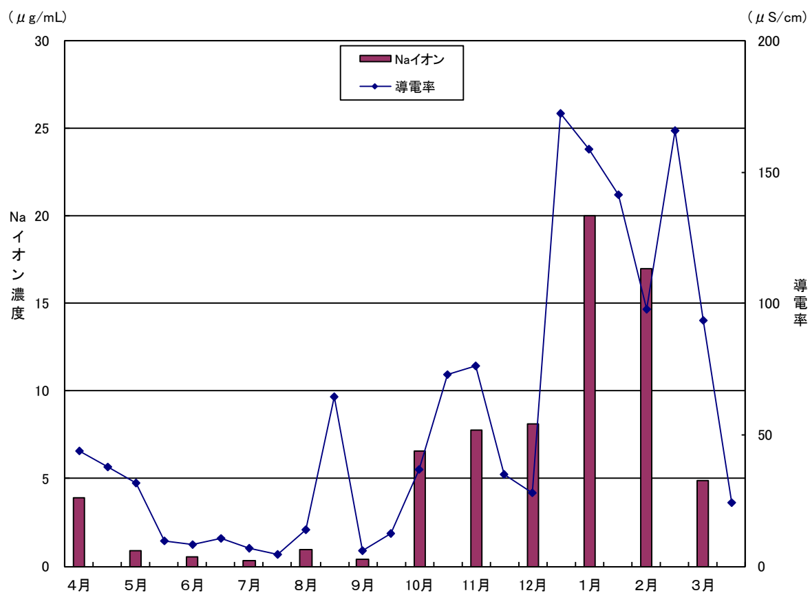
図 1-39 降水の導電率とNaイオン濃度の推移（令和2年度） （4～12月は山王、1～3月は八橋で調査）
