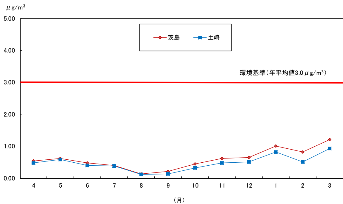
図1-36 ベンゼンの測定結果(令和2年度)
