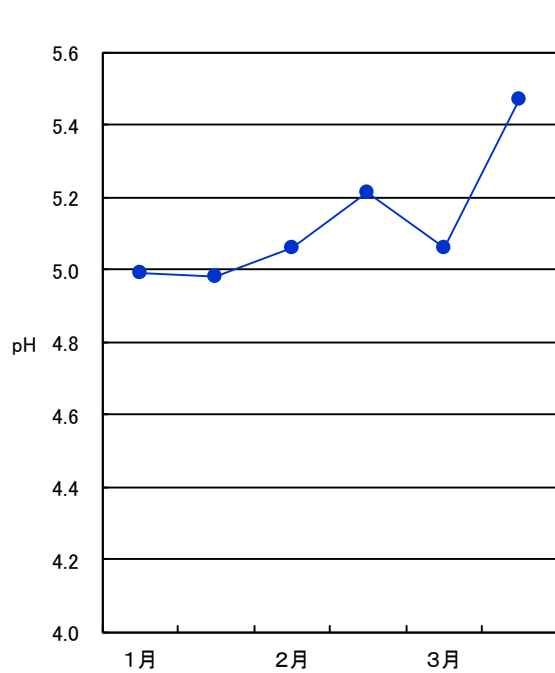
図 1-40 降雪のpHの推移（令和2年度）
