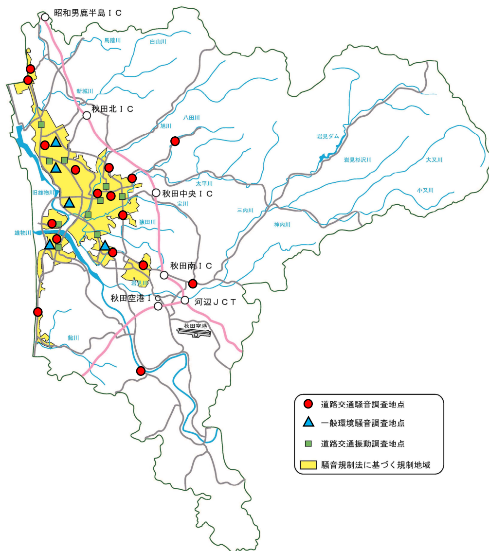
図3-1 騒音・振動状況調査地点図 (令和2年度)
