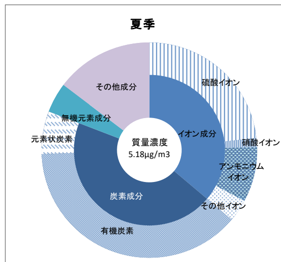
図1-29 PM2.5成分分析結果(夏季)(令和2年度)
