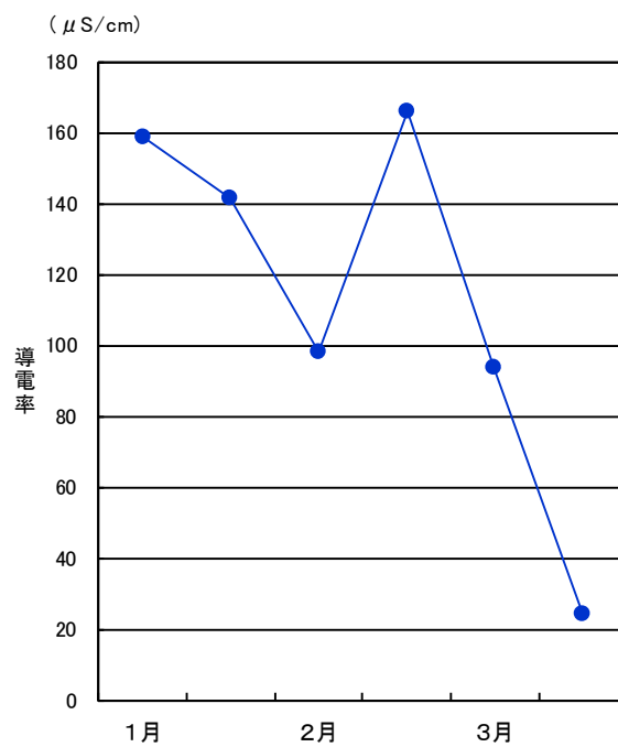
図 1-41 降雪の導電率の推移（令和2年度）
