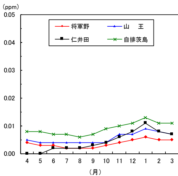
図1-14 二酸化窒素月平均値の変化(令和2年度)
