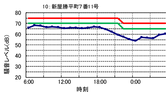
図3-2 道路交通騒音の24時間推移(1)(令和2年度)
