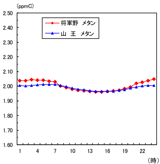
図1-34 メタンの時刻平均値の変化(令和2年度)
