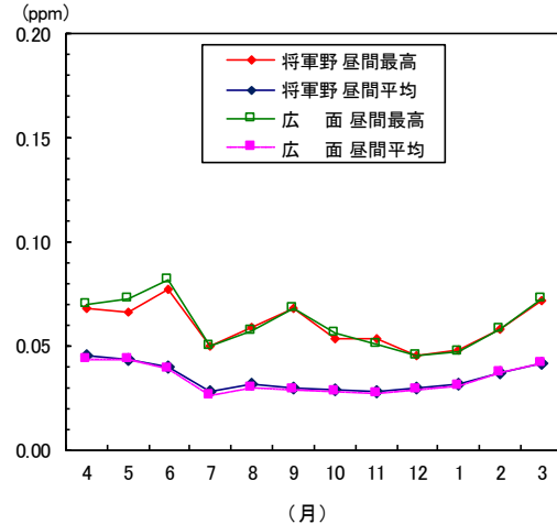
図1-23 光化学オキシダントの月平均値の変化（令和2年度）
