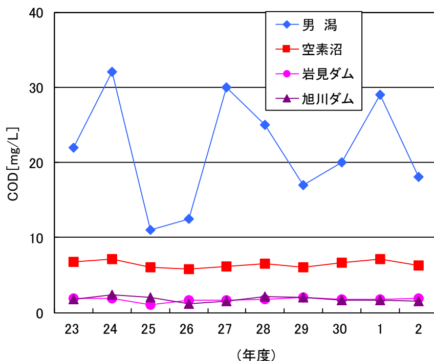
図 2-5 湖沼のCOD75%値の経年変化
