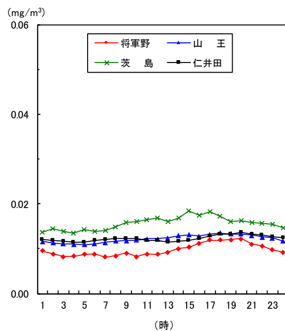
図1-18 浮遊粒子状物質の時刻平均値の変化 (令和2年度)
