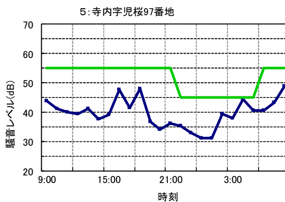
図 3－3 一般環境騒音の 24 時間推移 (令和2年度)
