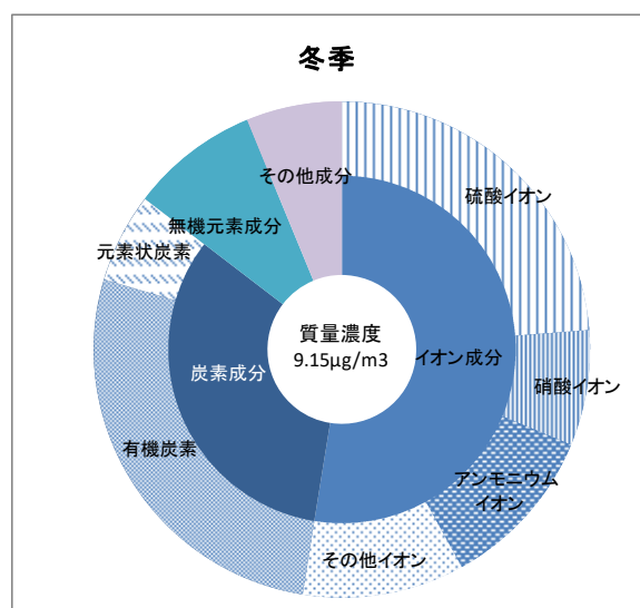
図1-31 PM2.5成分分析結果(冬季)(令和2年度)
