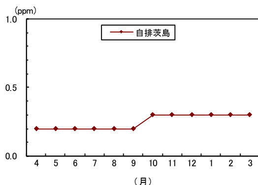
図1-20 一酸化炭素の月平均値の変化 （令和2年度）
