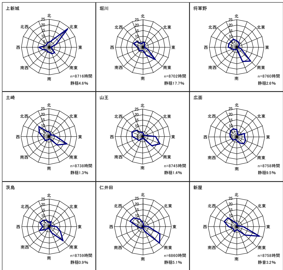
図1－4 風配図 (令和2年度)
