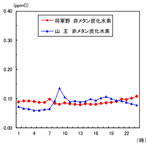
図1-33 非メタン炭化水素の時刻平均値の変化 (令和2年度)
