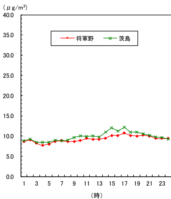
図1-27 微小粒子状物質の時刻平均値の変化 (令和2年度)
