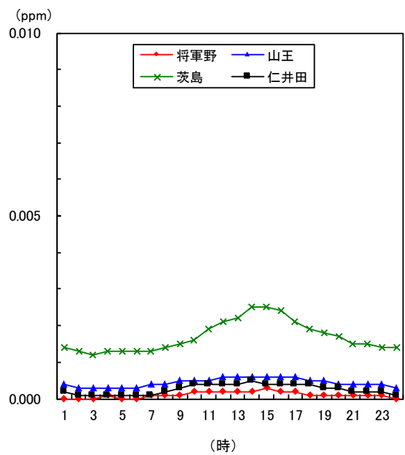
図1-9 二酸化硫黄時刻平均値の変化(令和2年度)
