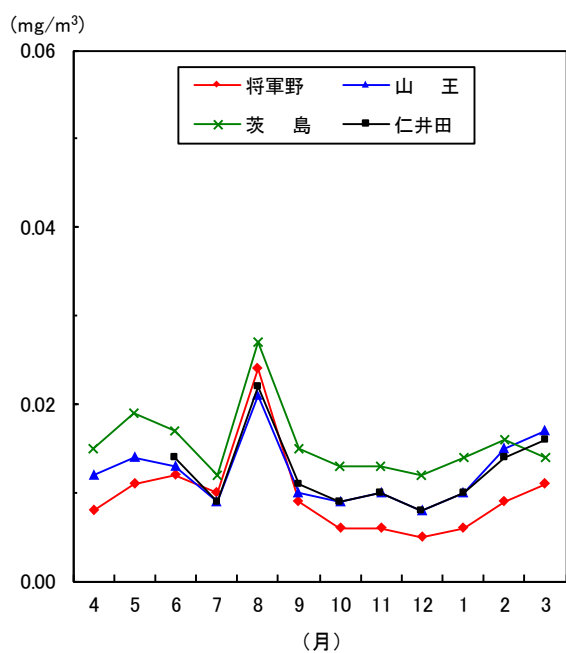
図1-17 浮遊粒子状物質の月平均値の変化(令和2年度)
