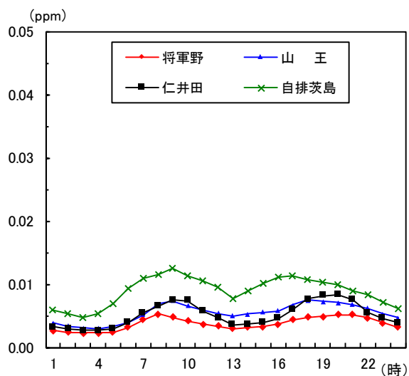
図1-13 二酸化窒素時刻平均値の変化(令和2年度)
