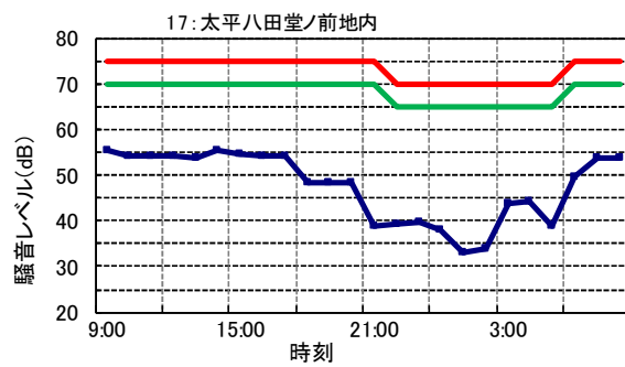
図 3 - 2 道路交通騒音の 24 時間推移 (2) (令和 2 年度)
