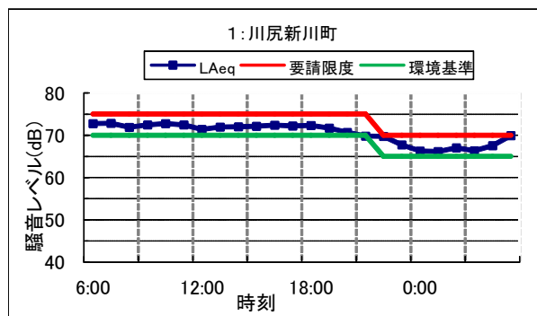
図 3-2 道路交通騒音の 24 時間推移
