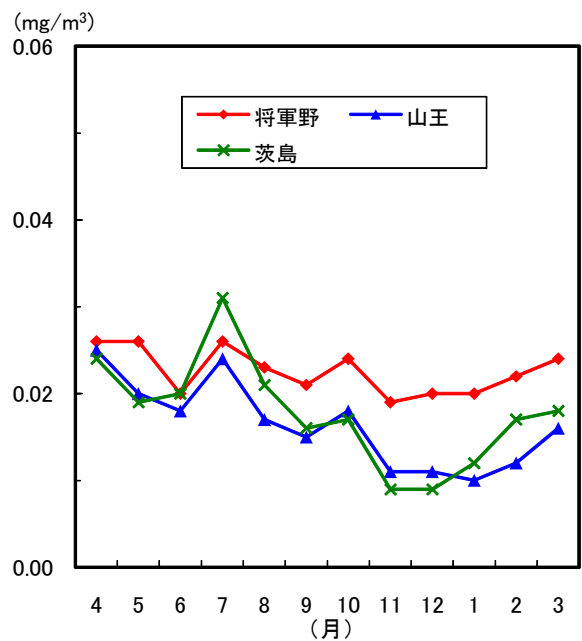
図1-17 浮遊粒子状物質の月平均値の変化 (平成20年度)
