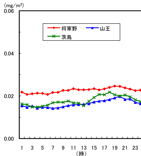
図1-18 浮遊粒子状物質の時刻平均値の変化 (平成20年度)
