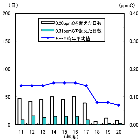
図 1－24 非メタン炭化水素の 6～9 時 3 時間平均値が指針値を超えた日数と年平均値の経年変化
