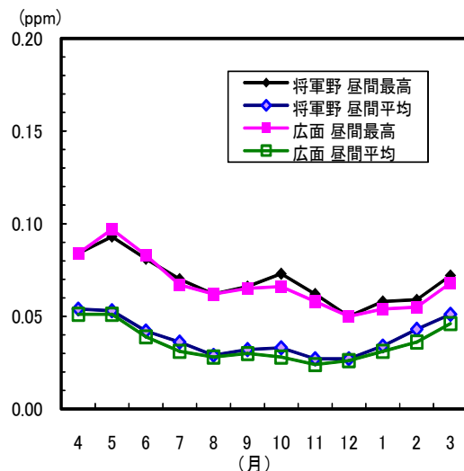
図1-23 光化学オキシダントの月平均値の変化（平成20年度）
