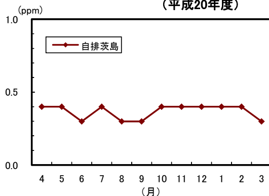
図1-20 一酸化炭素の月平均値の変化 (平成20年度)
