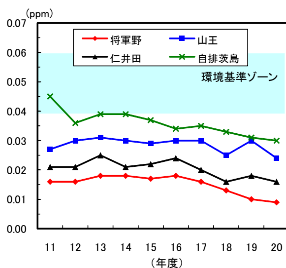
図1-13 二酸化窒素時刻平均値の変化 (平成20年度)
