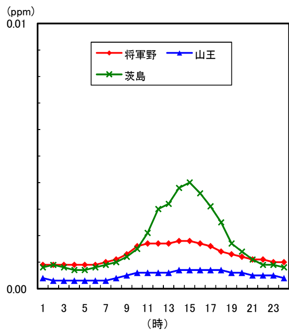
図1-9 二酸化いおう時刻平均値の変化(平成20年度)
