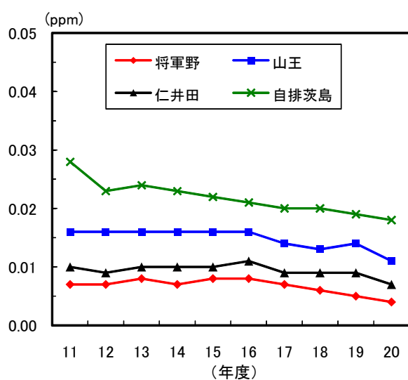
図1-12 一酸化窒素時刻平均値の変化 (平成20年度)
