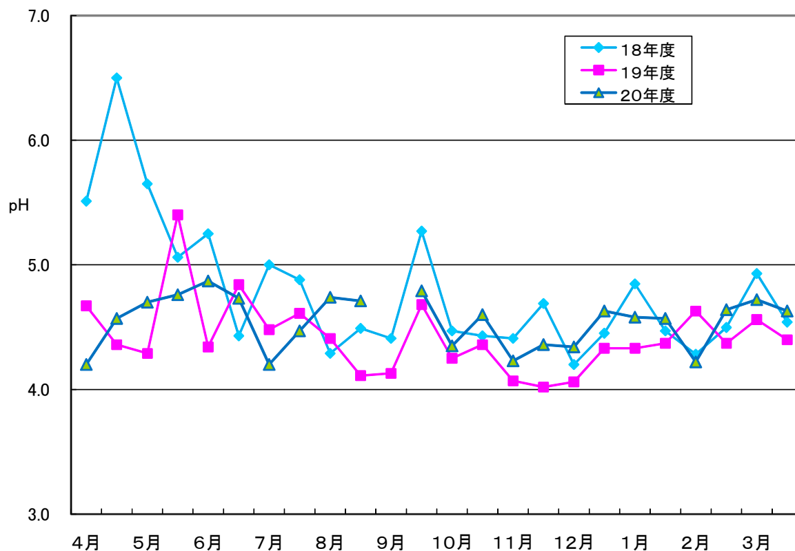
図1-30 酸性雨（山王）の加重平均値経年変化
