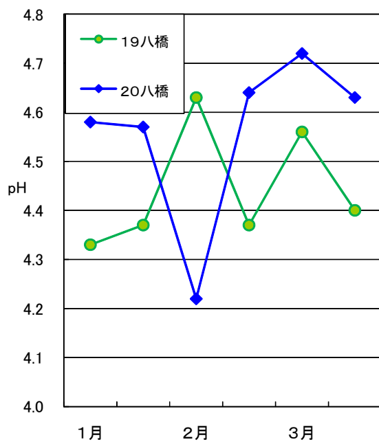
図1-32 降雪のpHの推移
