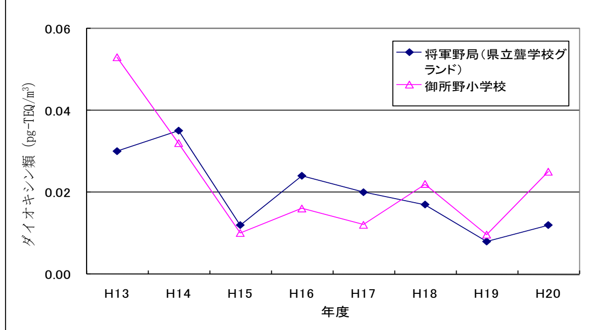
図5-1 大気中のダイオキシン類濃度の推移
