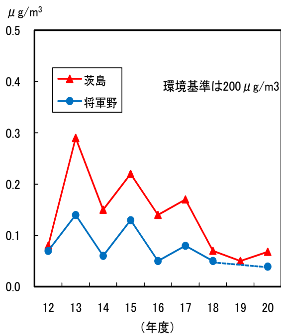
図1-27 トリクロロエチレンの年平均値の経年変化
