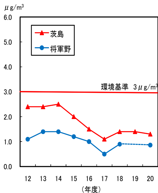
図1-26 ベンゼンの年平均値の経年変化
