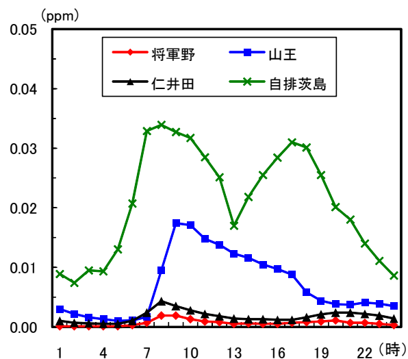
図1-14 二酸化窒素月平均値の変化 (平成20年度)
