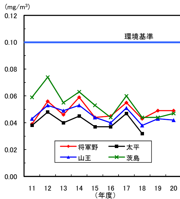
図1-16 浮遊粒子状物質の日平均値の年間2%除外値の経年変化
