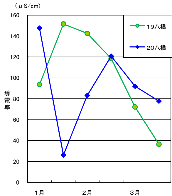
図1-33 降雪の導電率の推移
