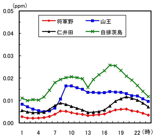
図1-13 二酸化窒素時刻平均値の変化 (平成20年度)
