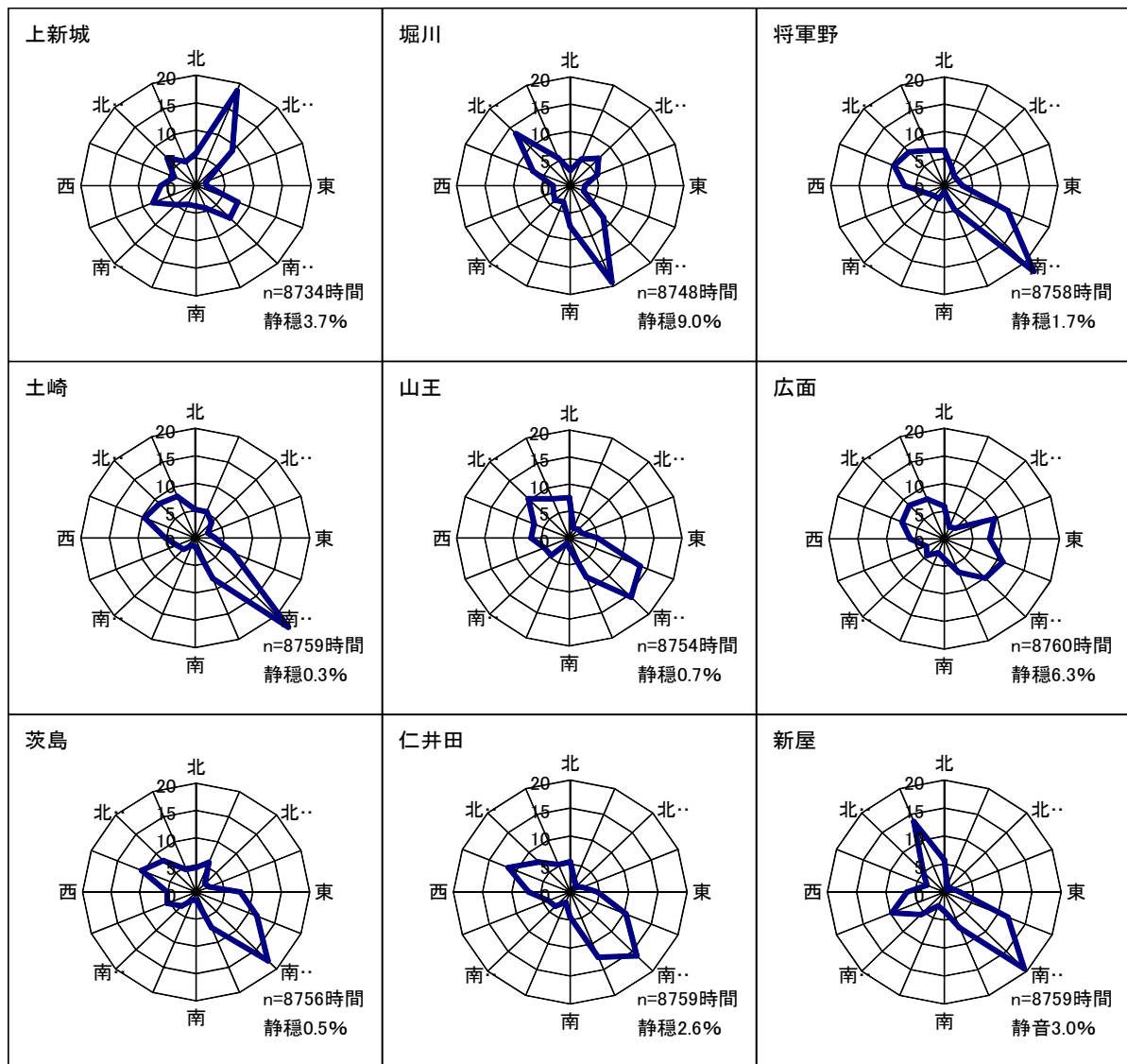
図1－4 風配図（平成20年度）
