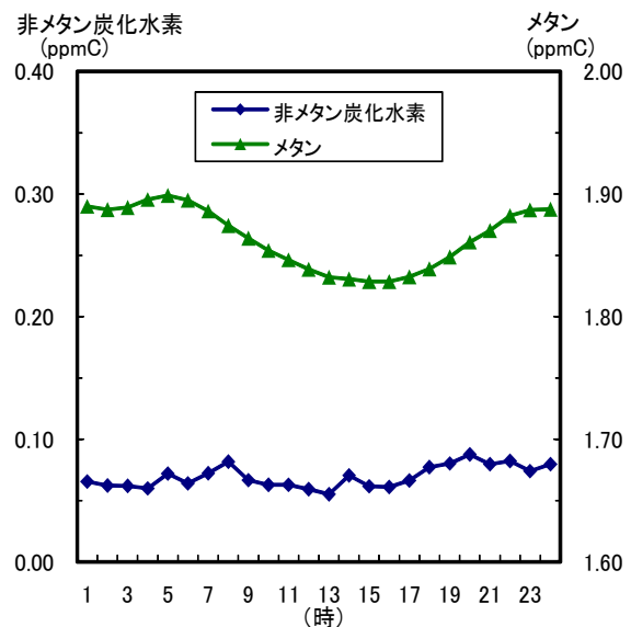
図 1－25 非メタン炭化水素とメタンの時刻平均値の変化(平成20年度)
