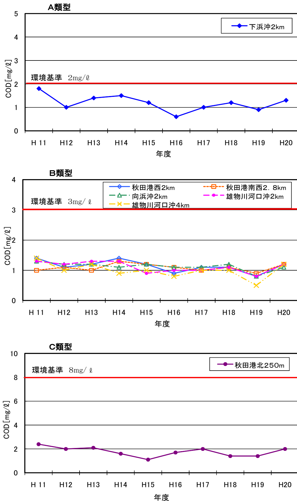
図 2-4 海域の COD75%値の経年変化
