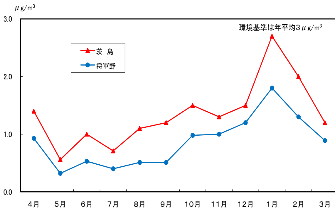
図1-28 ベンゼンの測定結果(平成20年度)
