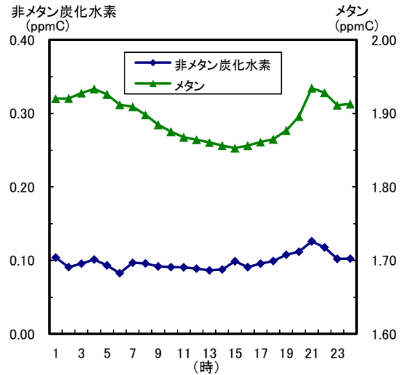
図 1－25 非メタン炭化水素とメタンの時刻平均値の変化(平成23年度)
