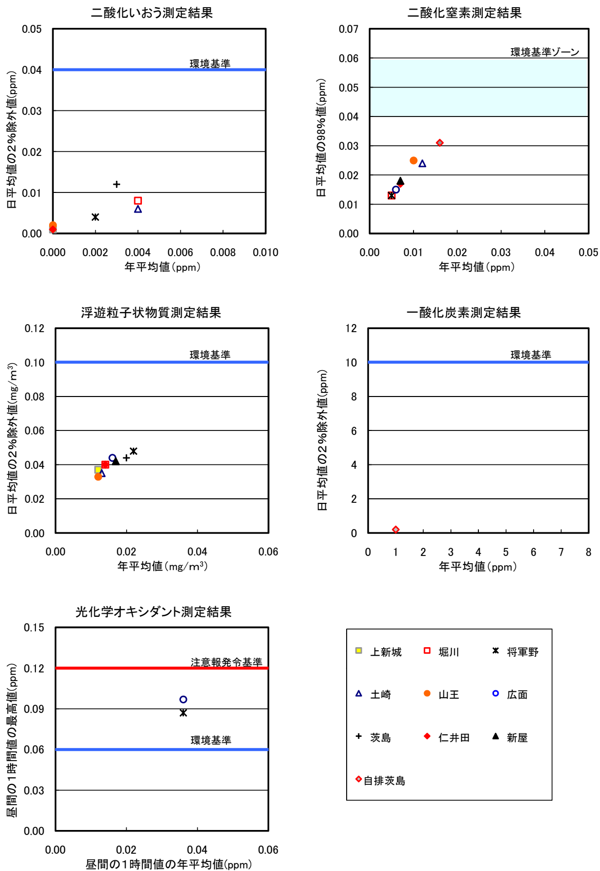
図1-3 大気環境基準の達成状況 (平成23年度)
