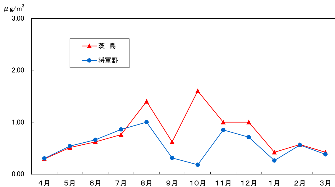
図1-28 ベンゼンの測定結果(平成23年度)
