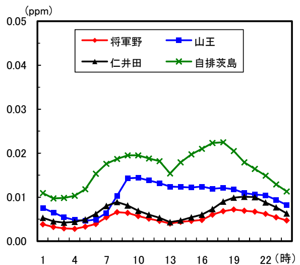
図1-13 二酸化窒素時刻平均値の変化 (平成23年度)
