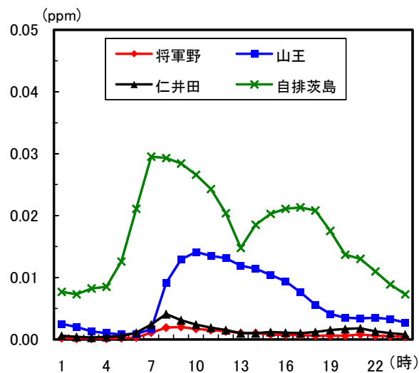
図1-12 一酸化窒素時刻平均値の変化 (平成23年度)
