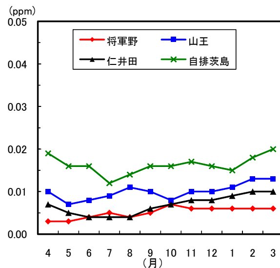
図1-14 二酸化窒素月平均値の変化 (平成23年度)
