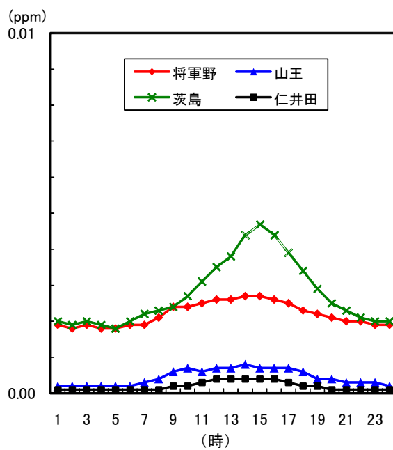
図1-9 二酸化いおう時刻平均値の変化(平成23年度)
