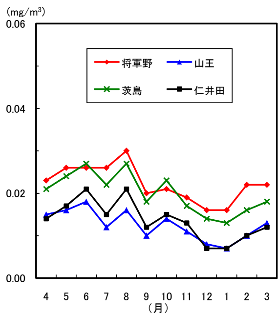
図1-17 浮遊粒子状物質の月平均値の変化 (平成23年度)
