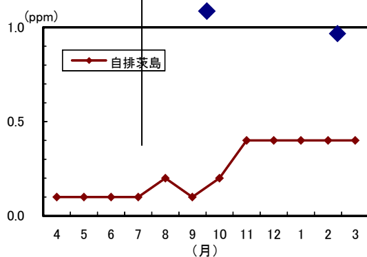
図 1－20 一酸化炭素の月平均値の変化 （平成 23 年度）
