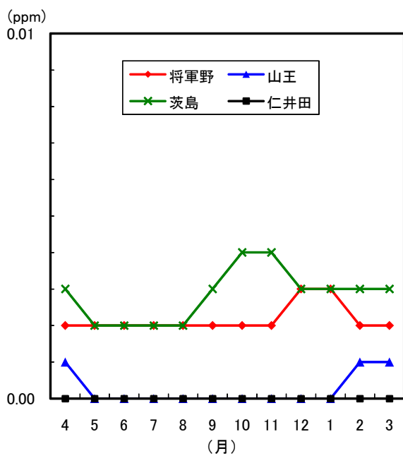
図1-8 二酸化いおう月平均値の変化(平成23年度)
