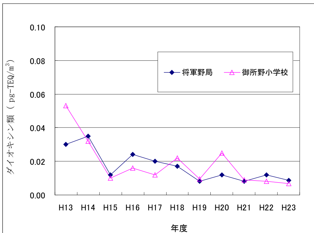
図 5－1 大気中のダイオキシン類濃度の推移
