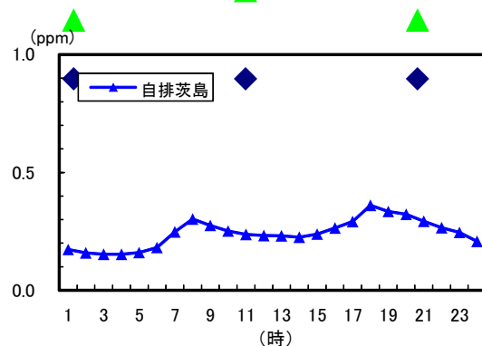
図 1－21 一酸化炭素の時刻平均値の変化 （平成 23 年度）
