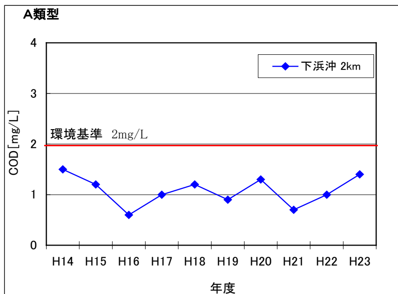
図 2-4 海域のCOD75%値の経年変化
