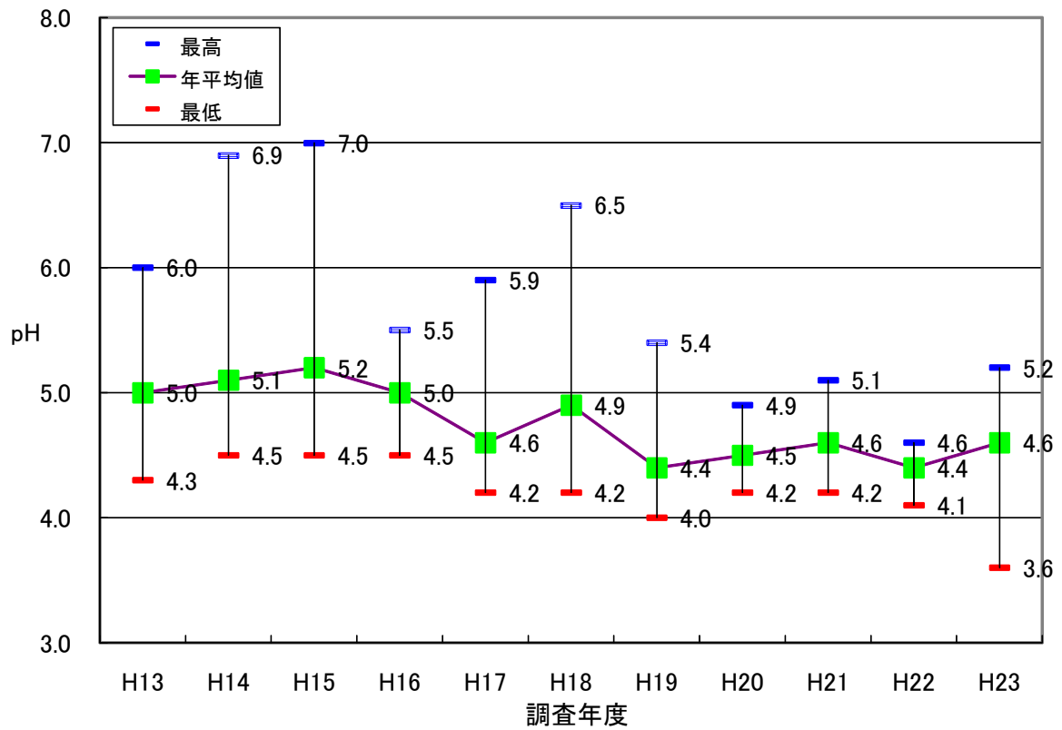
図1-30 酸性雨（山王）の平均値経年変化
