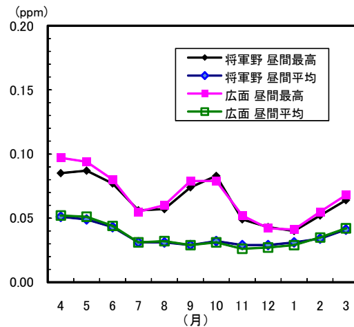
図 1-23 光化学オキシダントの月平均値の変化（平成 23 年度）
