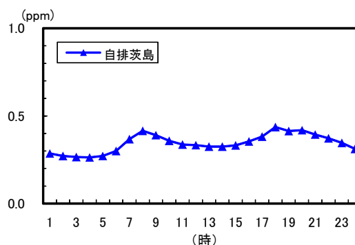
図1－21 一酸化炭素の時刻平均値の変化 （平成24年度）
