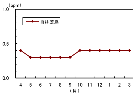
図1－20 一酸化炭素の月平均値の変化 （平成24年度）
