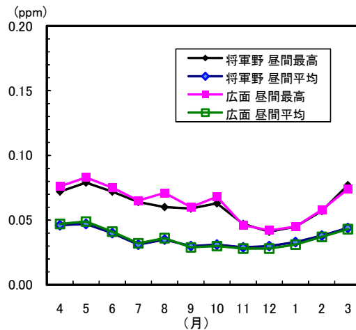
図1-23 光化学オキシダントの月平均値の変化（平成24年度）
