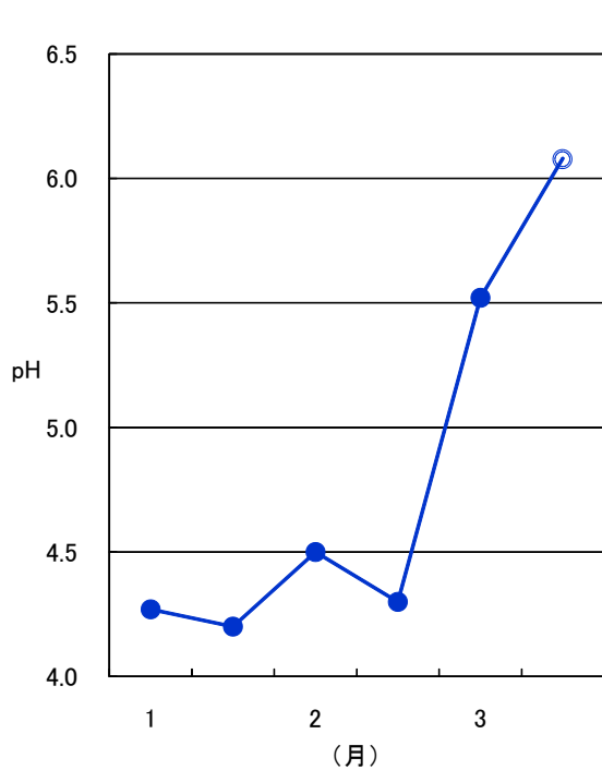
図1-36 降雪のpHの推移
