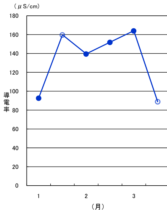
図1-37 降雪の導電率の推移
