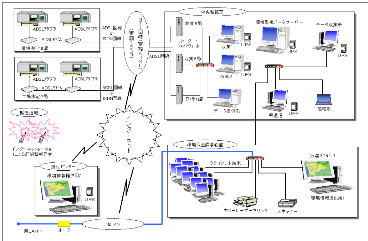
図 1-2 テレメータシステムの概要
