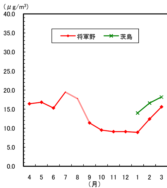
図1-26 微小粒子状物質の月平均値の変化 (平成24年度)
