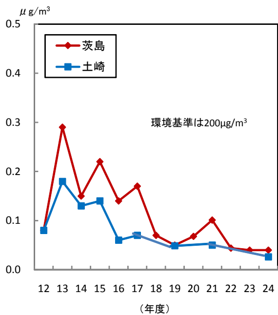
図1-31 トリクロロエチレンの年平均値の経年変化
