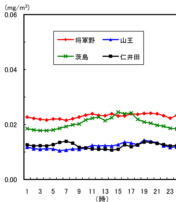
図1-18 浮遊粒子状物質の時刻平均値の変化 (平成24年度)
