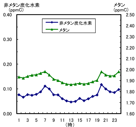
図 1－29 非メタン炭化水素とメタンの時刻平均値の変化（平成 24 年度）
