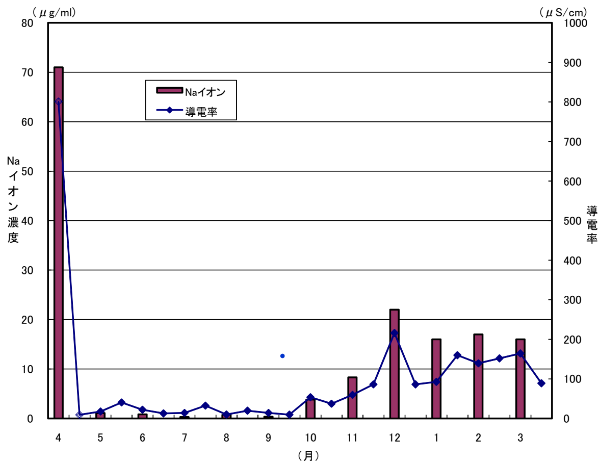
図1-35 降水の導電率とNaイオン濃度の推移（4～12月は山王、1～3月は八橋で調査）
