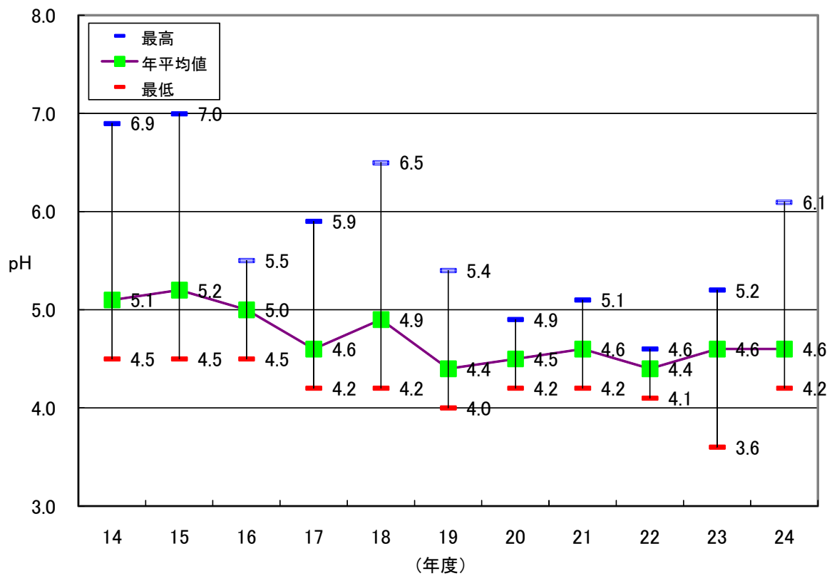
図1－34 酸性雨（山王）の平均値経年変化
