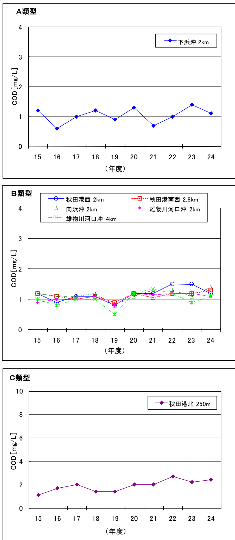
図 2 - 4 海域のCOD75%値の経年変化
