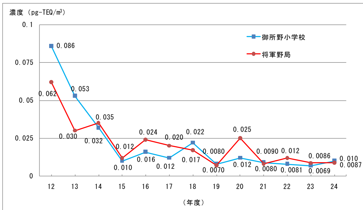
図 5－1 大気中のダイオキシン類濃度の推移
