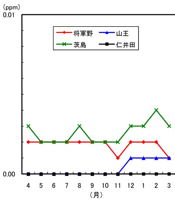
図1-8 二酸化いおう月平均値の変化(平成24年度)
