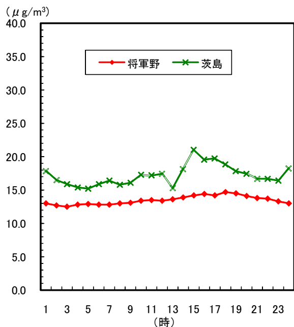
図1-27 微小粒子状物質の時刻平均値の変化 (平成24年度)
