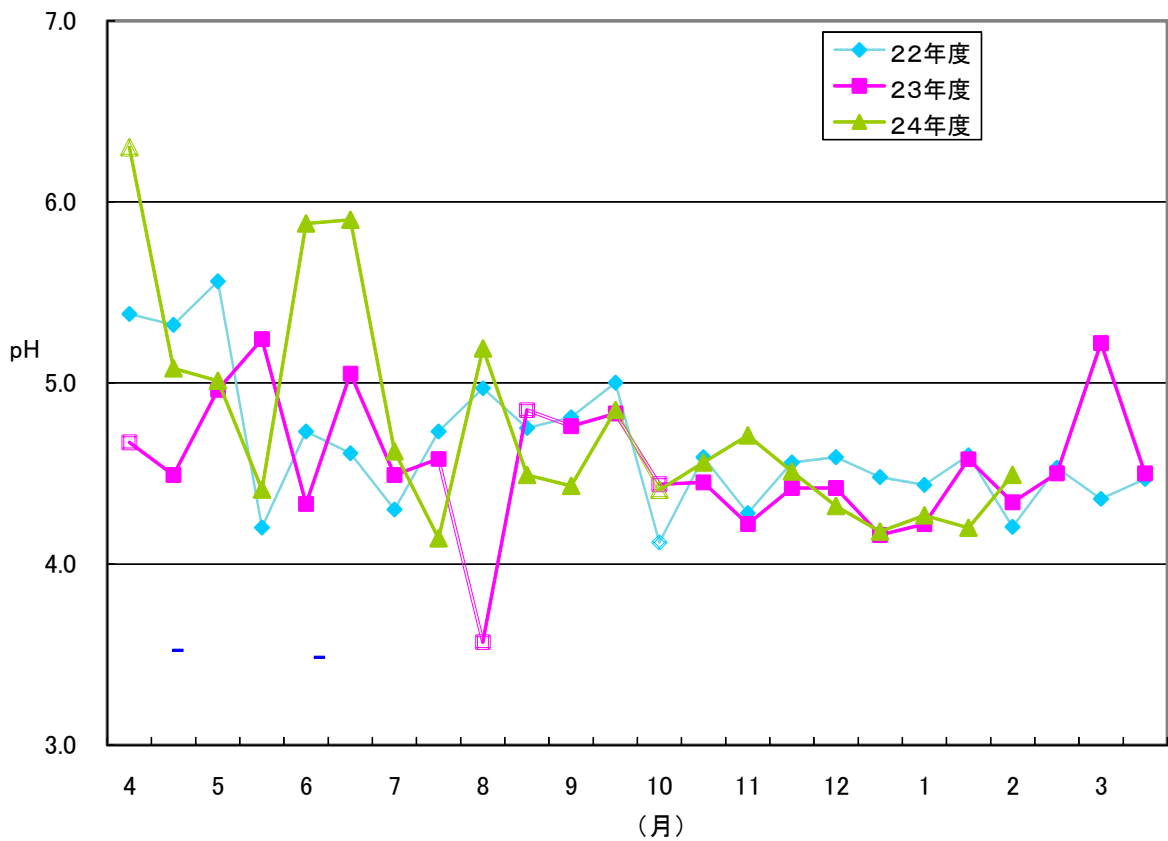
図 1－33 酸性雨・酸性雪の pH（月平均値）の変化（4～12月は山王、1～3月は八橋で調査）
