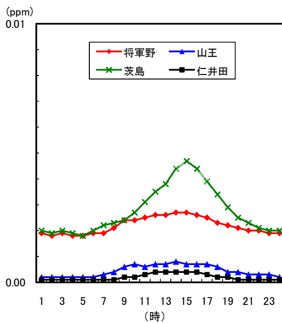
図1-9 二酸化いおう時刻平均値の変化(平成24年度)
