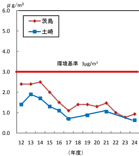
図1-30 ベンゼンの年平均値の経年変化
