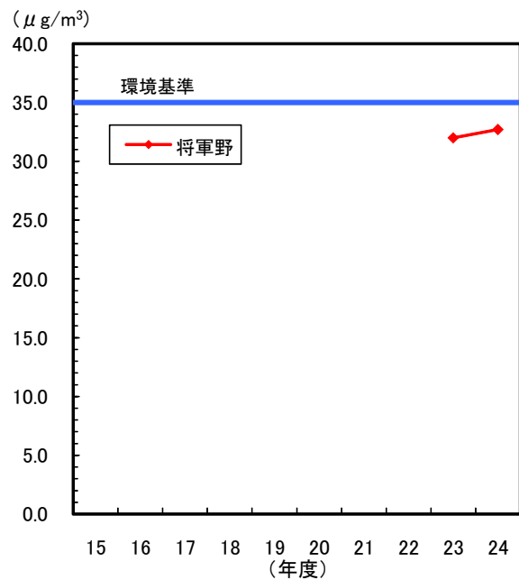
図1-25 微小粒子状物質の日平均値の年間2%除外値の経年変化
