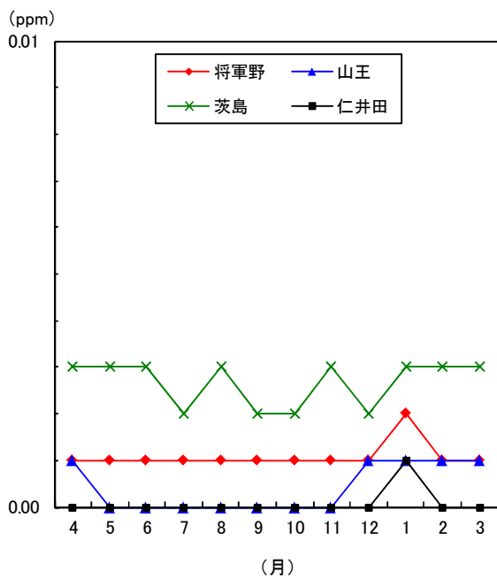
図1-8 二酸化いおう月平均値の変化(平成25年度)
