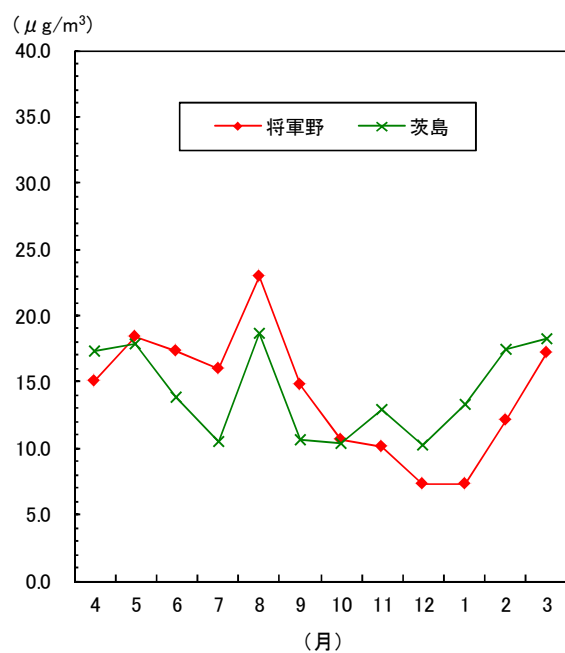
図1-26 微小粒子状物質の月平均値の変化 (平成25年度)
