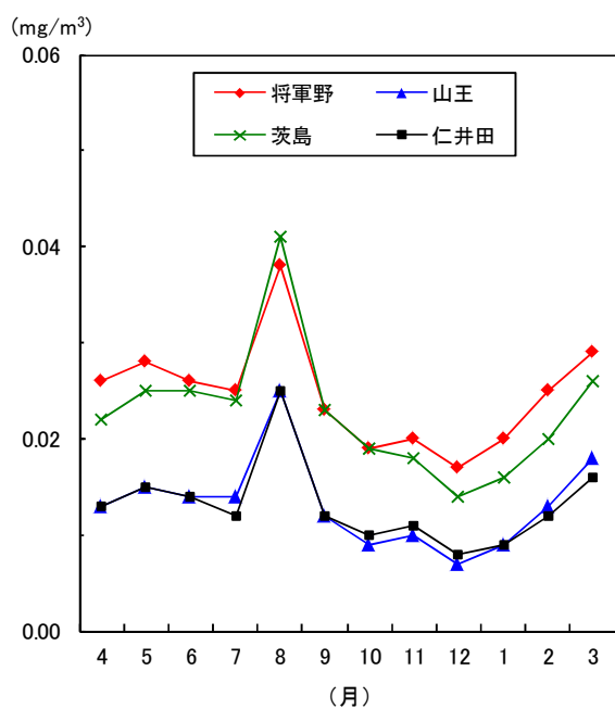
図1-17 浮遊粒子状物質の月平均値の変化 (平成25年度)
