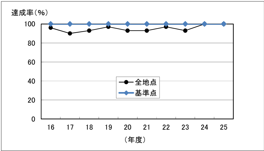
図 2-2 河川の BOD 75% 値による環境基準達成率（秋田市調査分）
