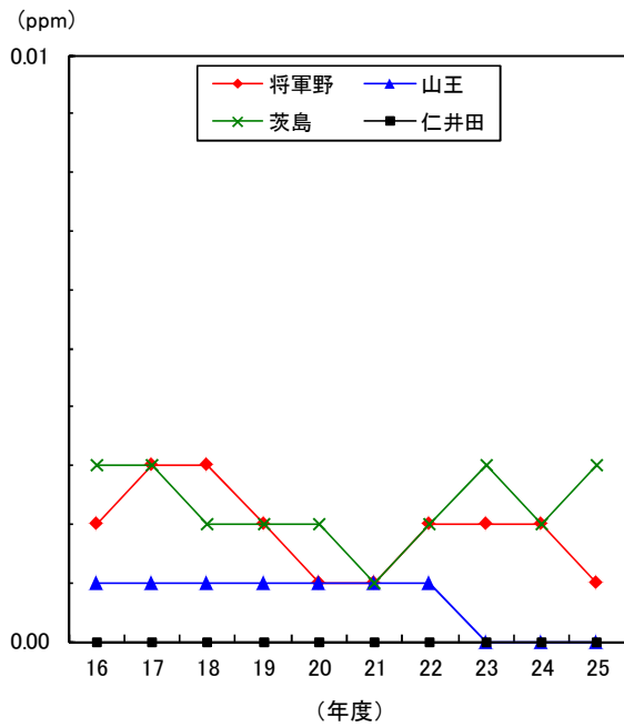
図1-6 二酸化いおう年平均値の経年変化
