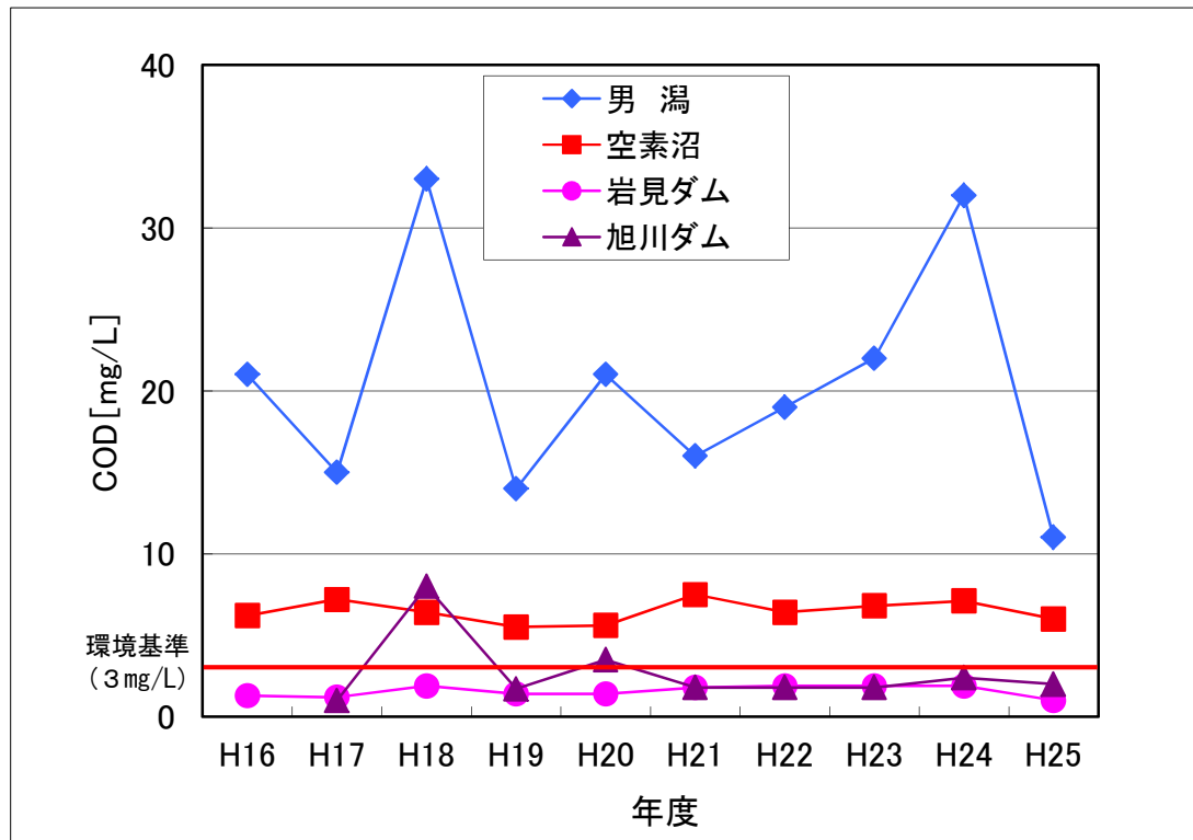
図 2－5 湖沼のCOD75%値の経年変化
