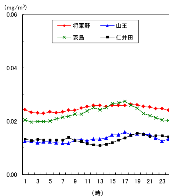
図1-18 浮遊粒子状物質の時刻平均値の変化 (平成25年度)
