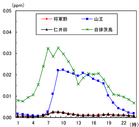
図1-12 一酸化窒素時刻平均値の変化 (平成25年度)
