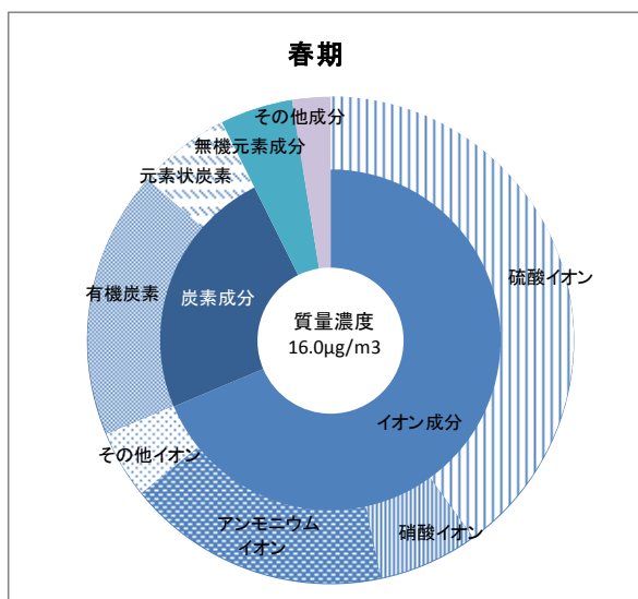
図1-28 PM2.5成分分析結果(春期) (平成25年度)
