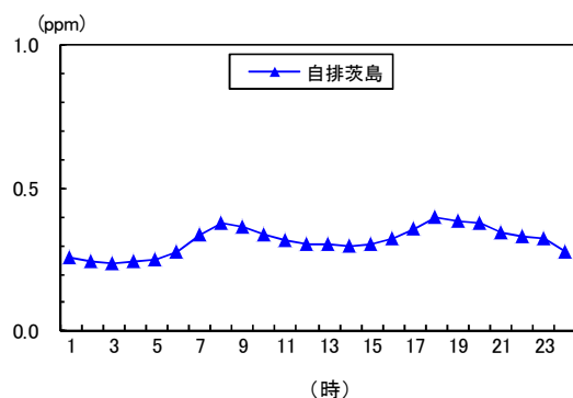
図1-21 一酸化炭素の時刻平均値の変化 （平成25年度）
