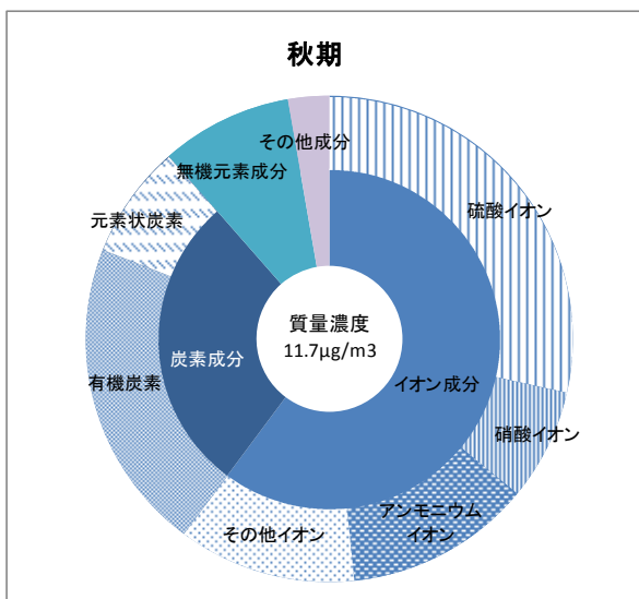
図1-30 PM2.5成分分析結果(秋期) (平成25年度)
