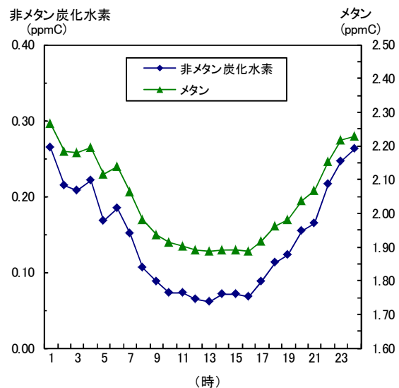
図 1-33 非メタン炭化水素とメタンの時刻平均値の変化（平成 25 年度）
