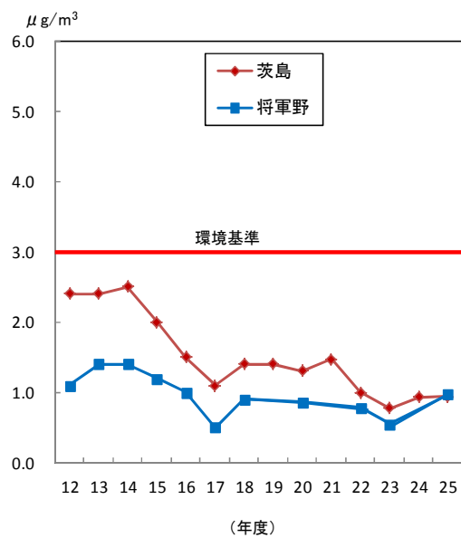
図1-34 ベンゼンの年平均値の経年変化
