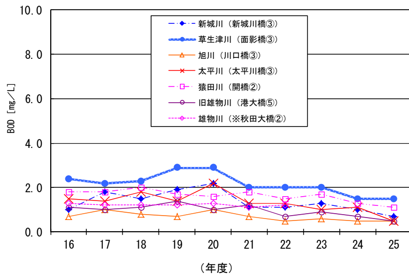
市内主要河川のBOD(75%値)の推移
