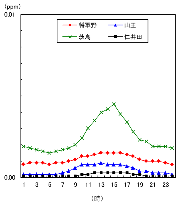
図1-9 二酸化いおう時刻平均値の変化(平成25年度)
