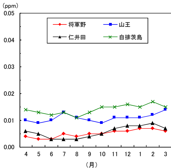
図1-14 二酸化窒素月平均値の変化 (平成25年度)
