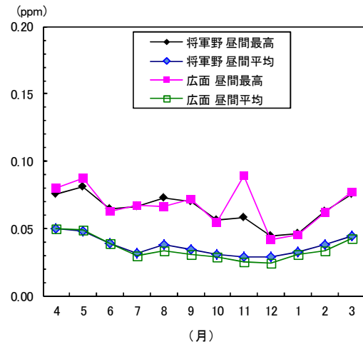
図1-23 光化学オキシダントの月平均値の変化（平成25年度）
