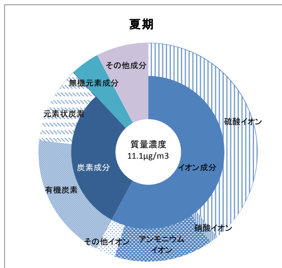
図1-29 PM2.5成分分析結果(夏期) (平成25年度)
