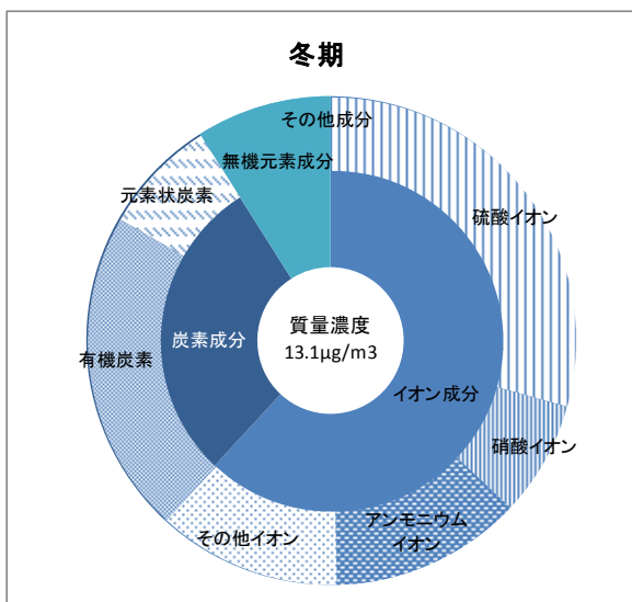
図1-31 PM2.5成分分析結果(冬期) (平成25年度)
