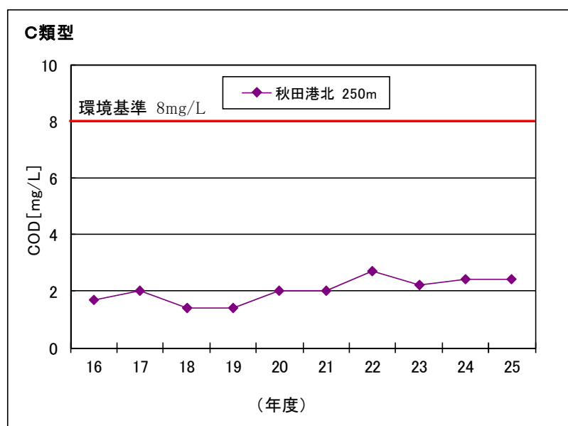
図 2 - 4 海域のCOD75%値の経年変化
