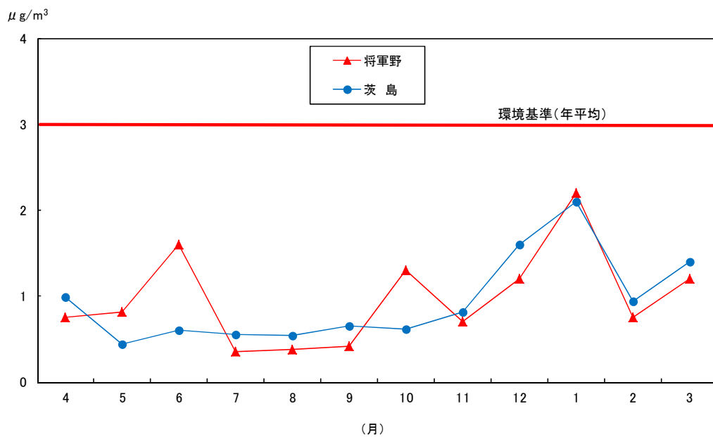
図1-36 ベンゼンの測定結果(平成25年度)
