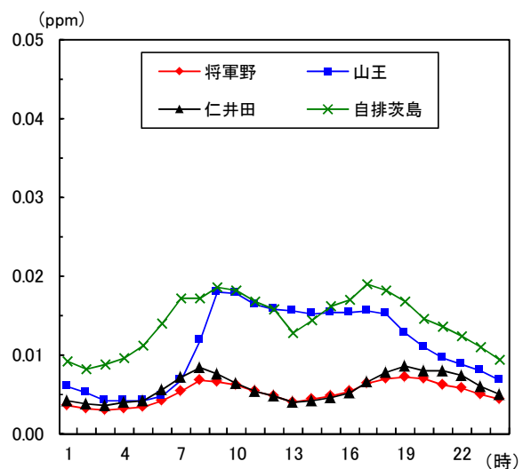
図1-13 二酸化窒素時刻平均値の変化 (平成25年度)
