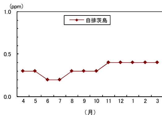
図1-20 一酸化炭素の月平均値の変化 （平成25年度）
