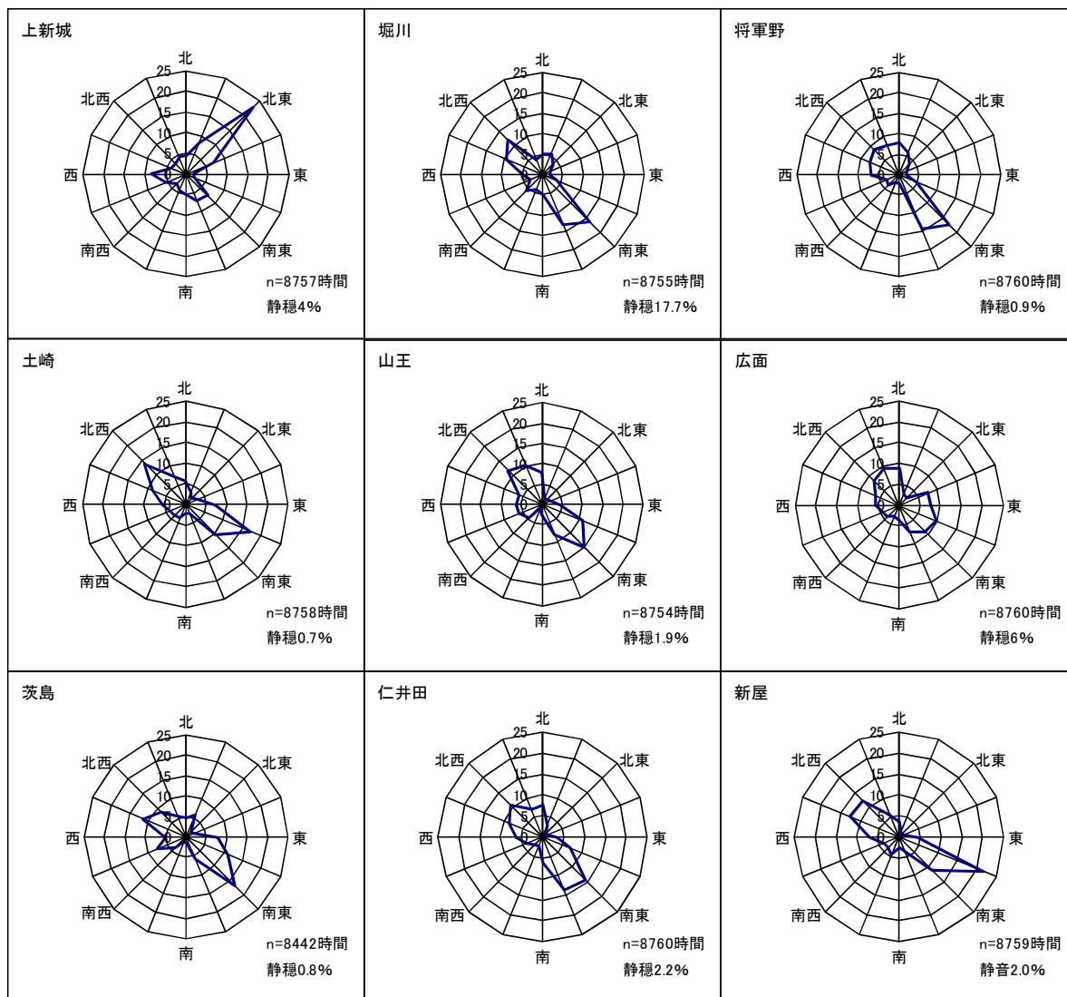
図1－4 風配図（平成25年度）
