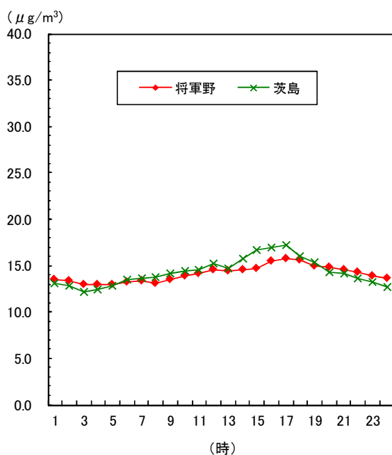
図1-27 微小粒子状物質の時刻平均値の変化 (平成25年度)
