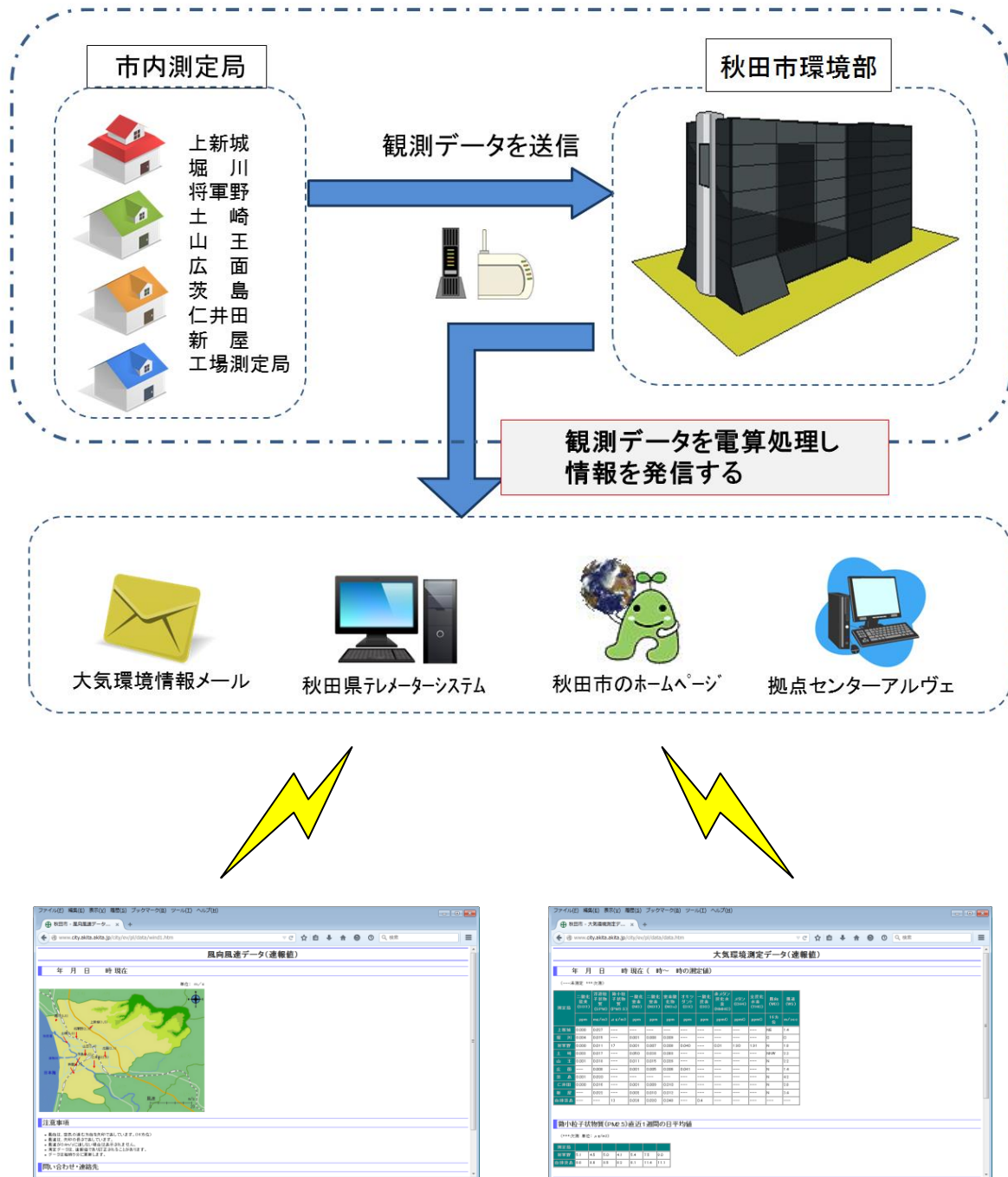
図 1-2 テレメーターシステムの概要
