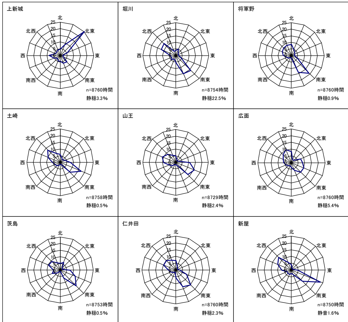
図 1－4 風配図（平成 28 年度）
