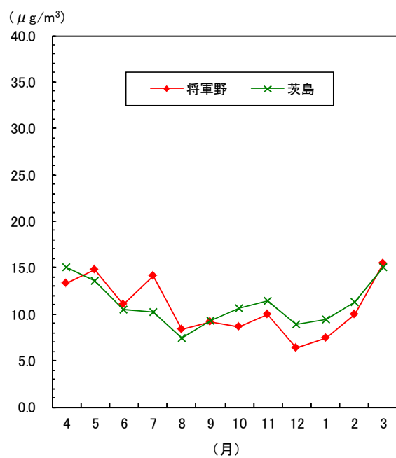
図1-26 微小粒子状物質の月平均値の変化 (平成29年度)
