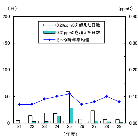
図 1-32 非メタン炭化水素の 6～9 時 3 時間平均値が指針値を超えた日数と年平均値の経年変化
