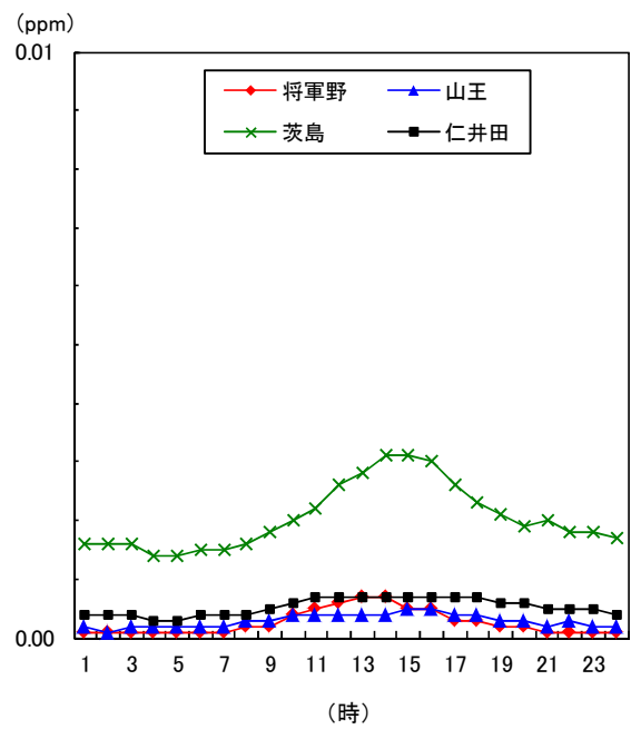
図1-9 二酸化硫黄時刻平均値の変化(平成29年度)
