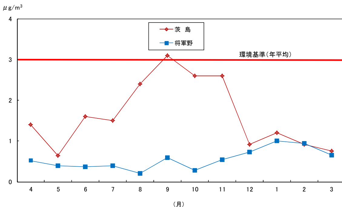
図1-36 ベンゼンの測定結果（平成29年度）
