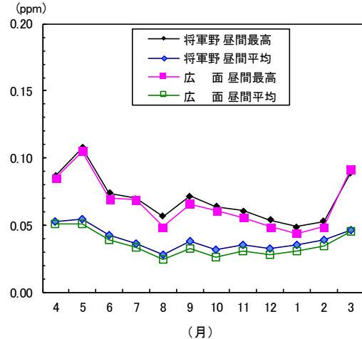
図1-23 光化学オキシダントの月平均値の変化（平成29年度）
