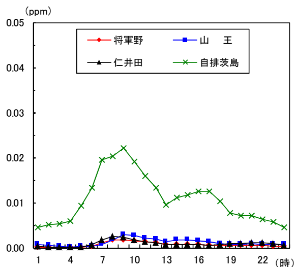
図1-12 一酸化窒素時刻平均値の変化 (平成29年度)
