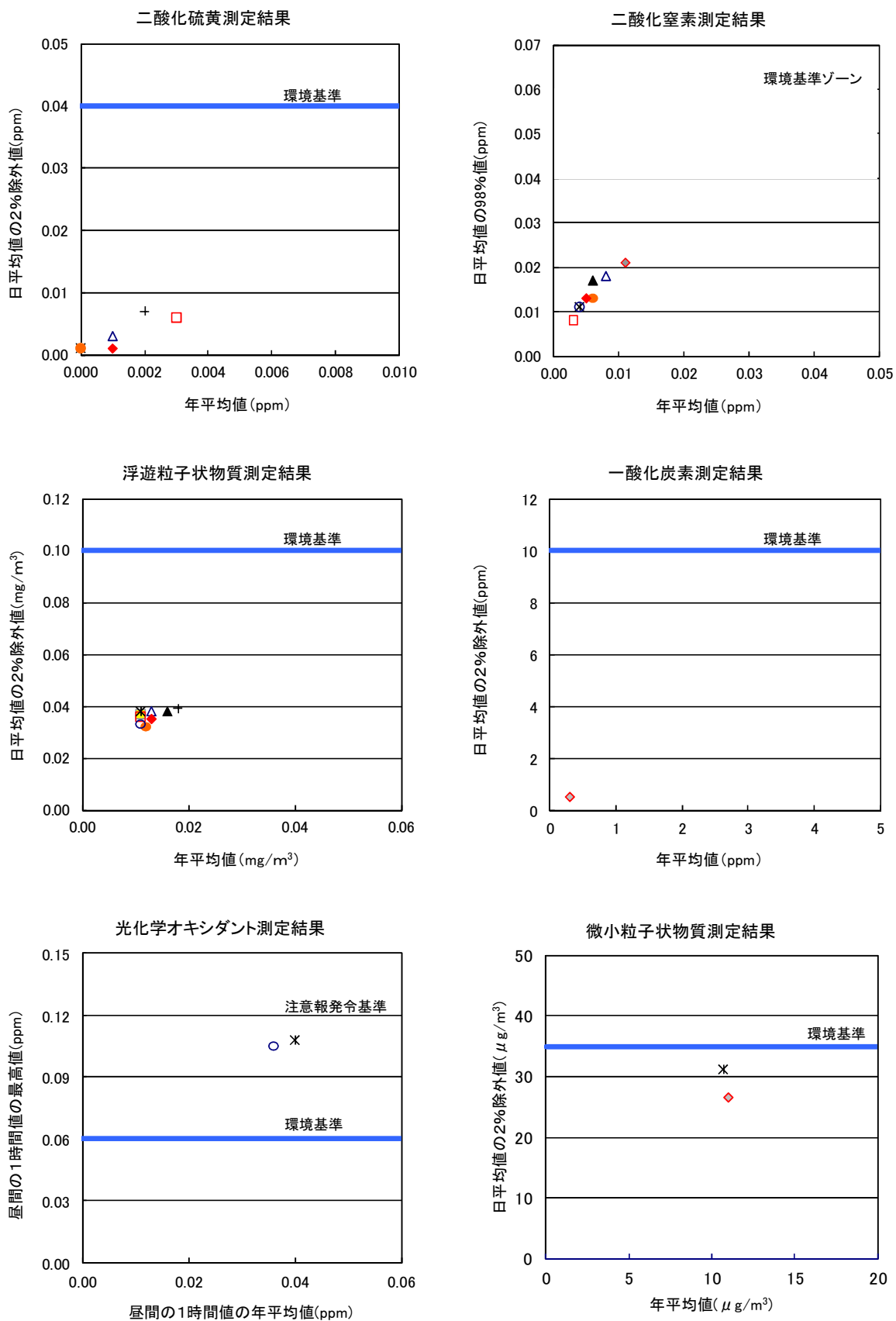
図1-3 大気環境基準の達成状況 (平成29年度)
