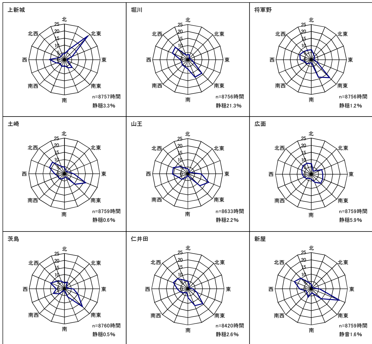
図1－4 風配図（平成29年度）
