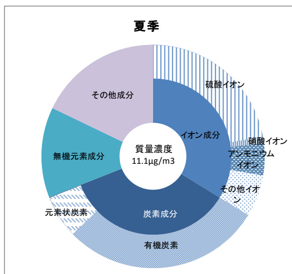
図1-29 PM2.5成分分析結果(夏季) (平成29年度)
