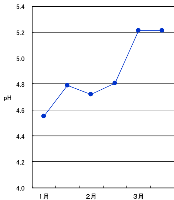
図 1-40 降雪のpHの推移（平成29年度）
