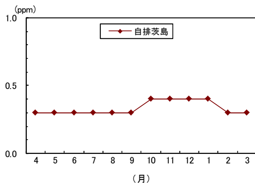
図1-20 一酸化炭素の月平均値の変化 （平成29年度）
