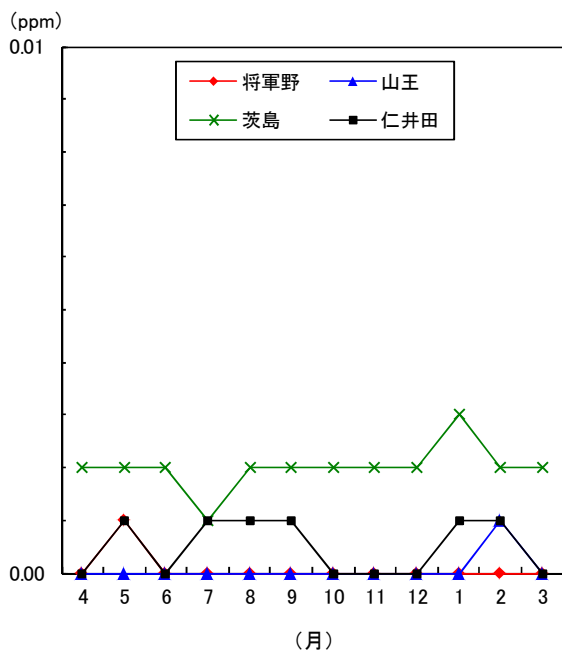
図1-8 二酸化硫黄月平均値の変化(平成29年度)
