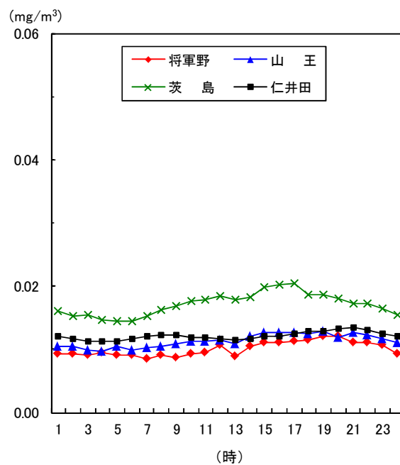
図1-18 浮遊粒子状物質の時刻平均値の変化 (平成29年度)
