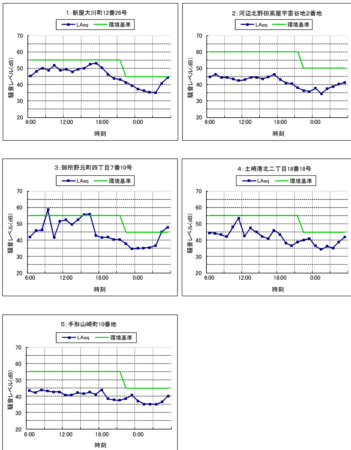
図 3-3 一般環境騒音の 24 時間推移
