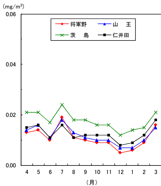
図1-17 浮遊粒子状物質の月平均値の変化 (平成29年度)
