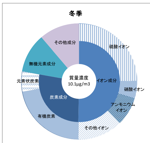
図1-31 PM2.5成分分析結果(冬季) (平成29年度)
