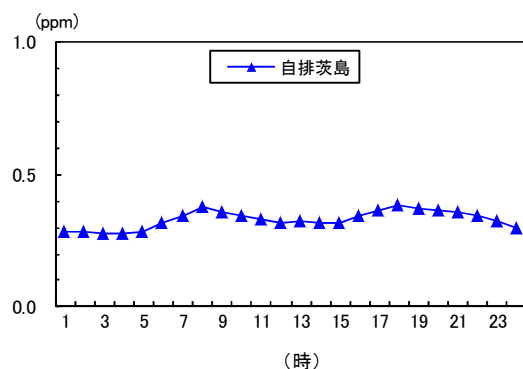
図1-21 一酸化炭素の時刻平均値の変化 （平成29年度）
