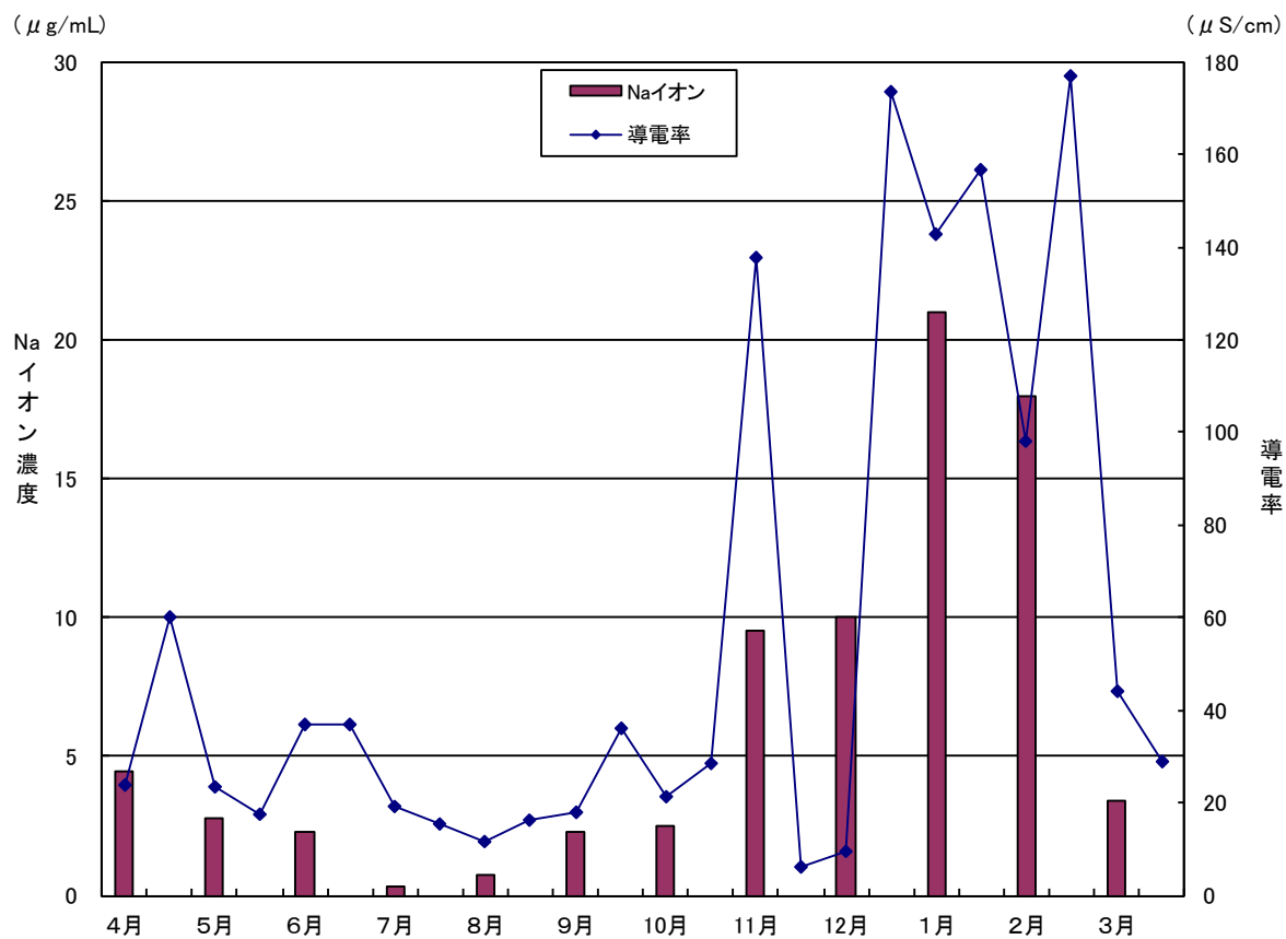
図 1-39 降水の導電率とNaイオン濃度の推移（平成29年度） （4～12月は山王、1～3月は八橋で調査）
