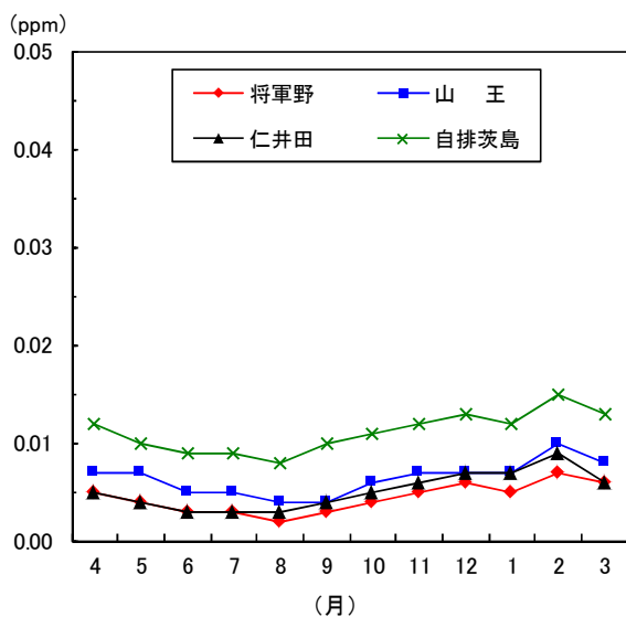
図1-12 一酸化窒素時刻平均値の変化 (平成29年度)
