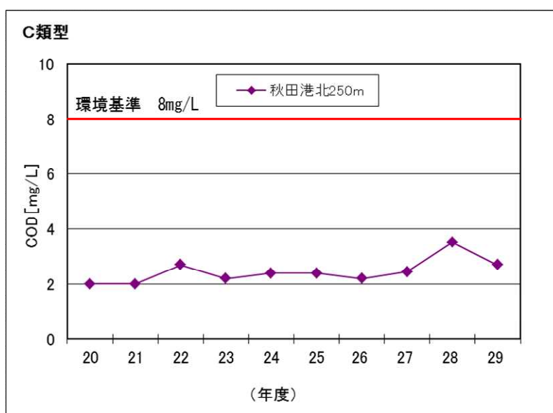
図 2 - 4 海域のCOD75%値の経年変化
