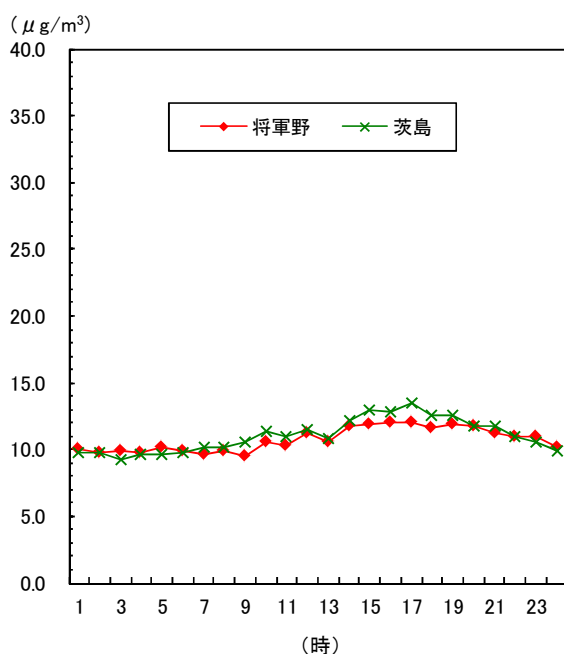
図1-27 微小粒子状物質の時刻平均値の変化 (平成29年度)
