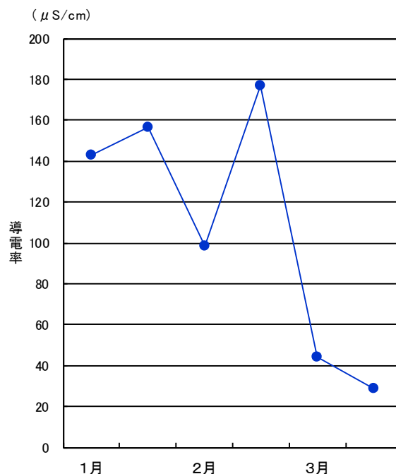
図 1-41 降雪の導電率の推移（平成29年度）
