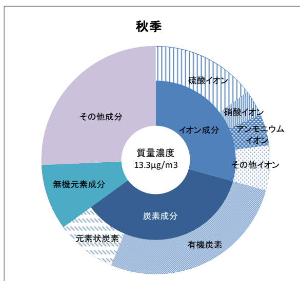
図1-30 PM2.5成分分析結果(秋季) (平成29年度)
