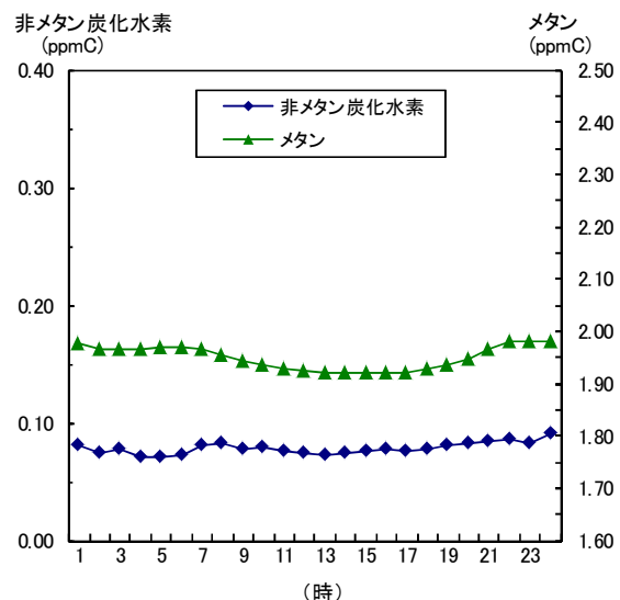
図 1-33 非メタン炭化水素とメタンの時刻平均値の変化（平成 29 年度）
