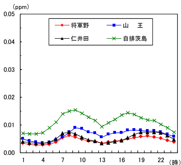
図1-13 二酸化窒素時刻平均値の変化 (平成29年度)
