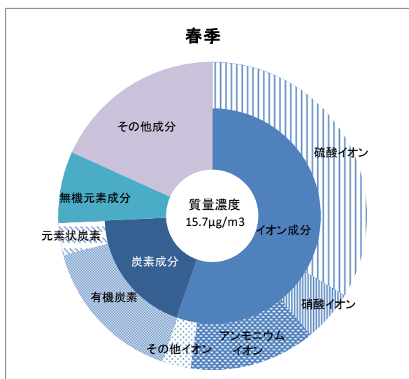
図1-28 PM2.5成分分析結果(春季) (平成29年度)
