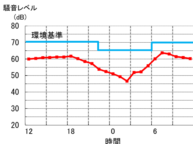
自動車交通騒音 (LAeq) 24 時間推移の一例 (広面字碇 76-1)
