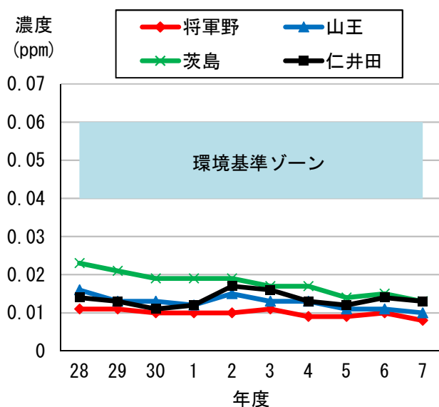
二酸化窒素の日平均値の経年変化
