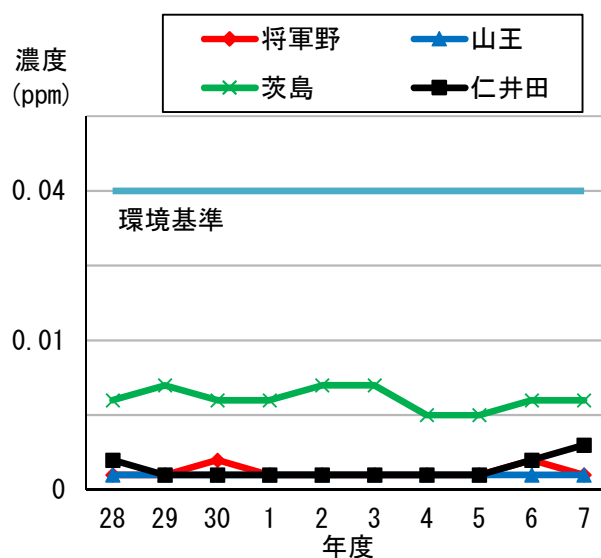
二酸化硫黄の日平均値の経年変化
