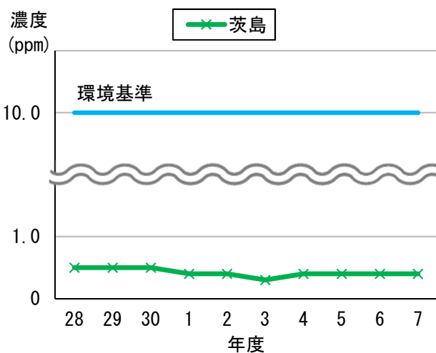
一酸化炭素の日平均値の経年変化
