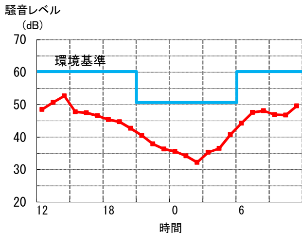
一般環境騒音 (LAeq) 24 時間推移の一例 (泉中央六丁目 3-1)
