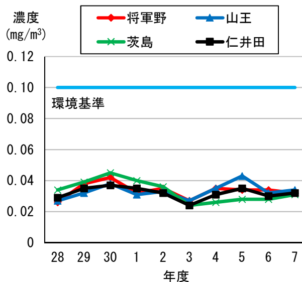
浮遊粒子状物質の日平均値の経年変化
