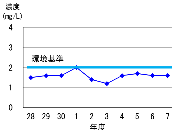
海域 COD 測定結果の経年変化（下浜沖）
