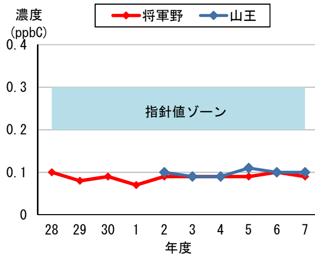
非メタン炭化水素の年平均値の経年変化
