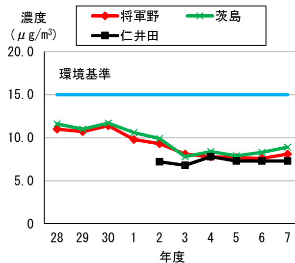
微小粒子状物質(PM2.5)の年平均値の経年変化
