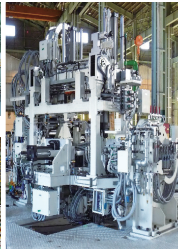
鑄造設備
