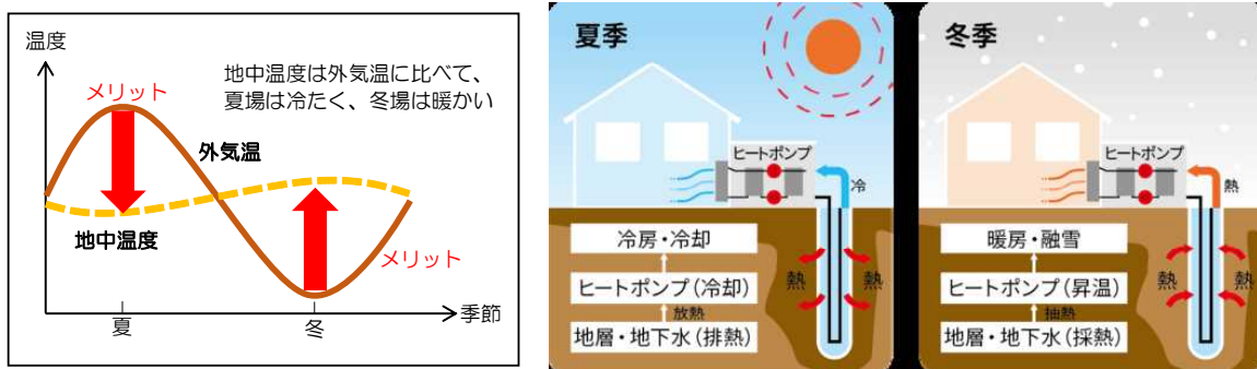
【図3-6】地中熱および地中熱ヒートポンプの概念図
