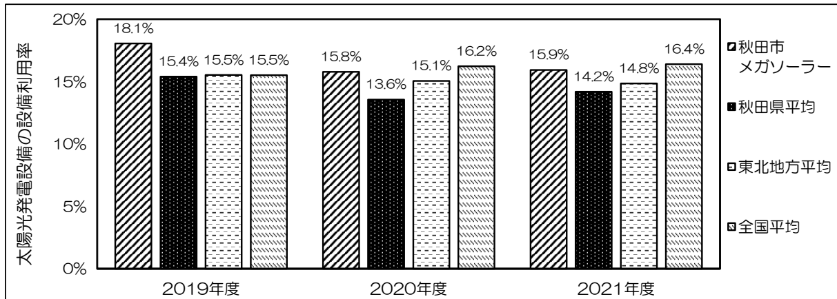
【図3-5】本市メガソーラーと県、東北地方および全国の太陽光発電設備の設備利用率比較 出典) 資源エネルギー庁 電力調査統計表から作成
