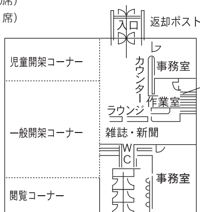
1 階平面図
