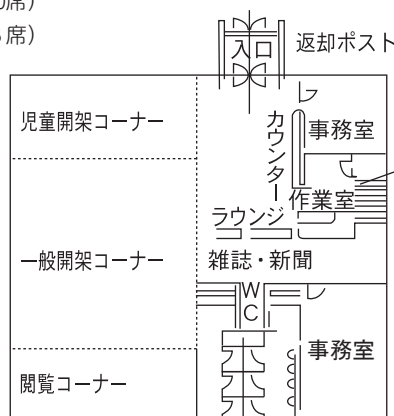
1 階平面図
