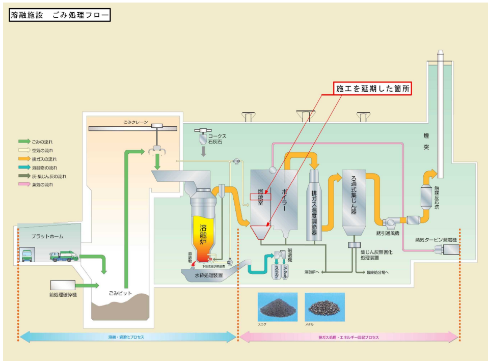
図1 ごみ処理全体フロー
