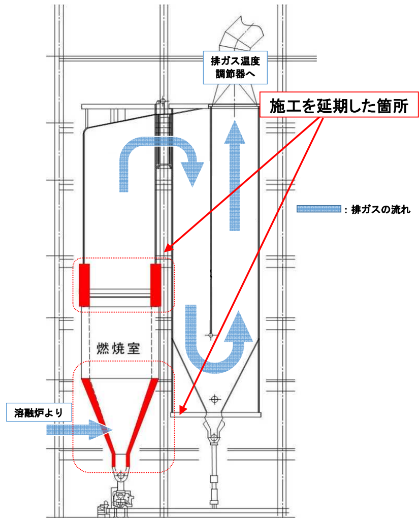
図2 燃焼室・ボイラー詳細
