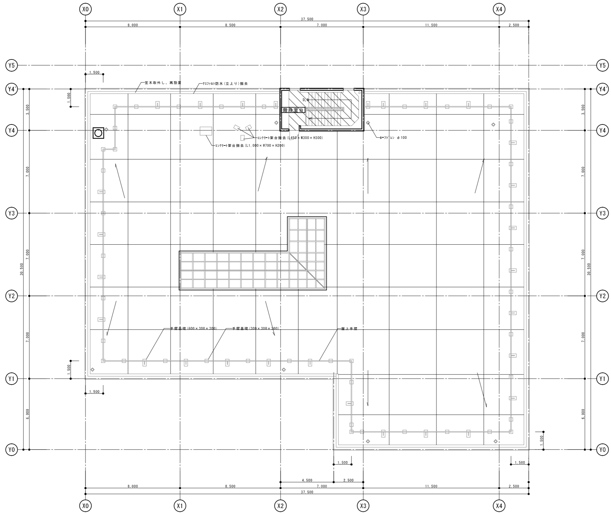
既存R階平面図 1/100
