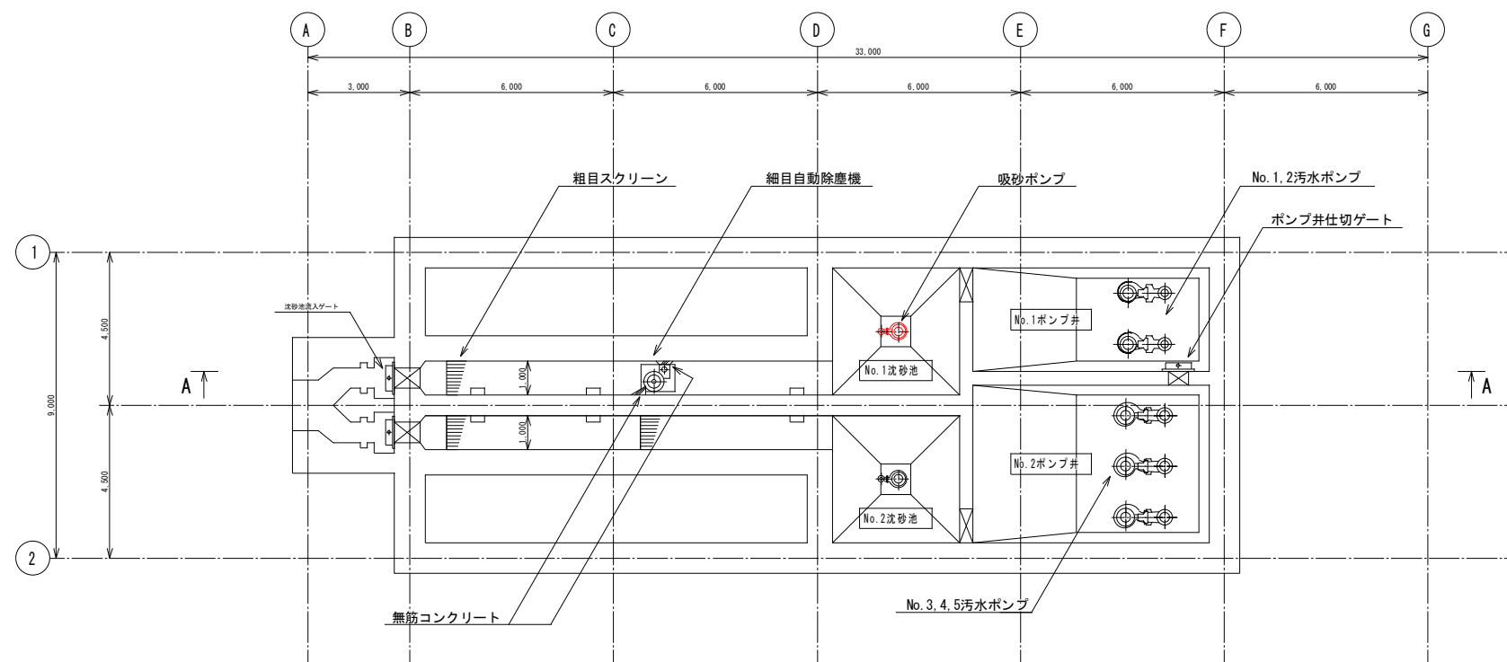
ポンプ井平面図
