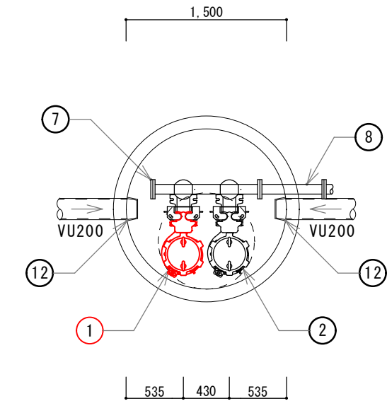
マンホール参考図（平面） S=NON
