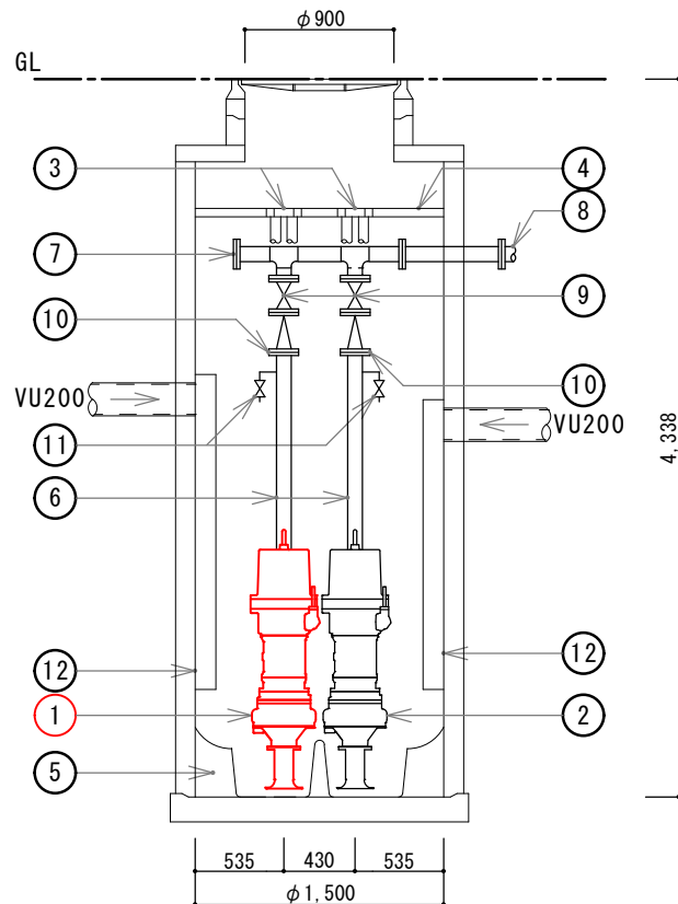
マンホール参考図（断面） S=NON
