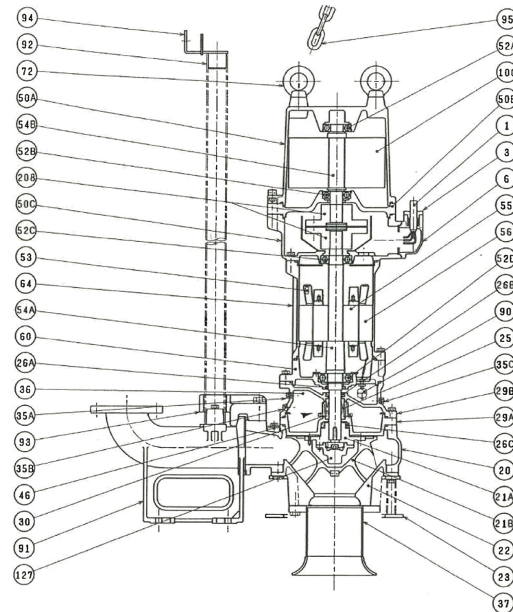
参考構造断面図 S=NON
