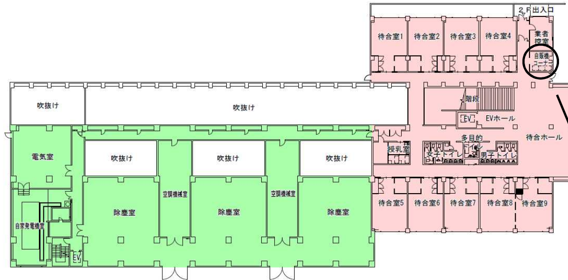
秋田市斎場2階平面図
