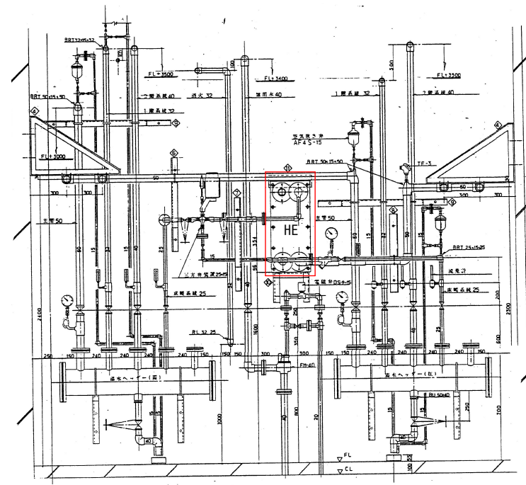
立面図
