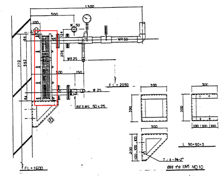
プレート式熱交換器 側面図
