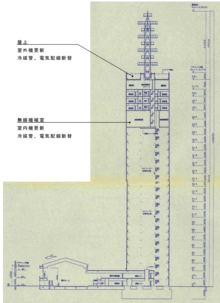
修繕図 S=NON
