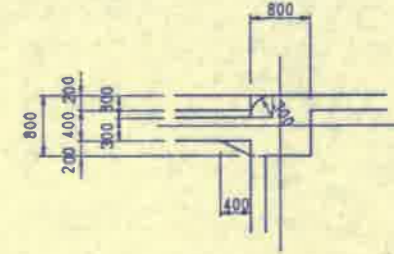
イ部詳細図 (縮尺 1/50)
