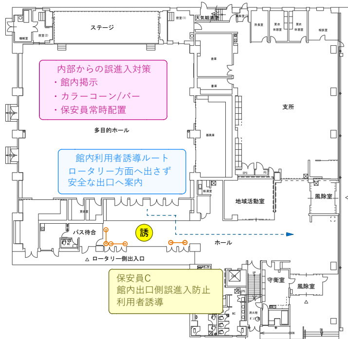
1 階平面図
