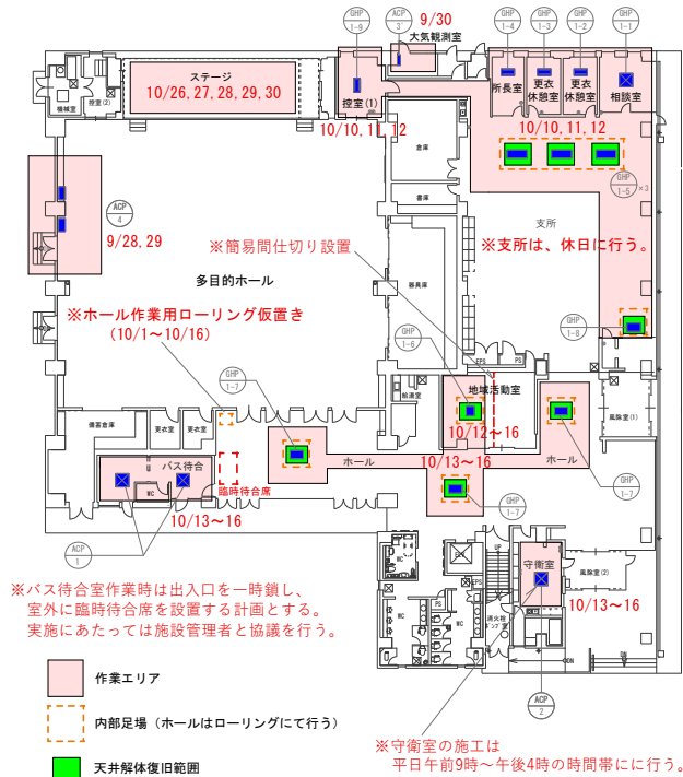
1 階平面図
