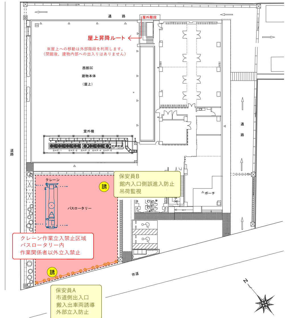
外部クレーン配置図
