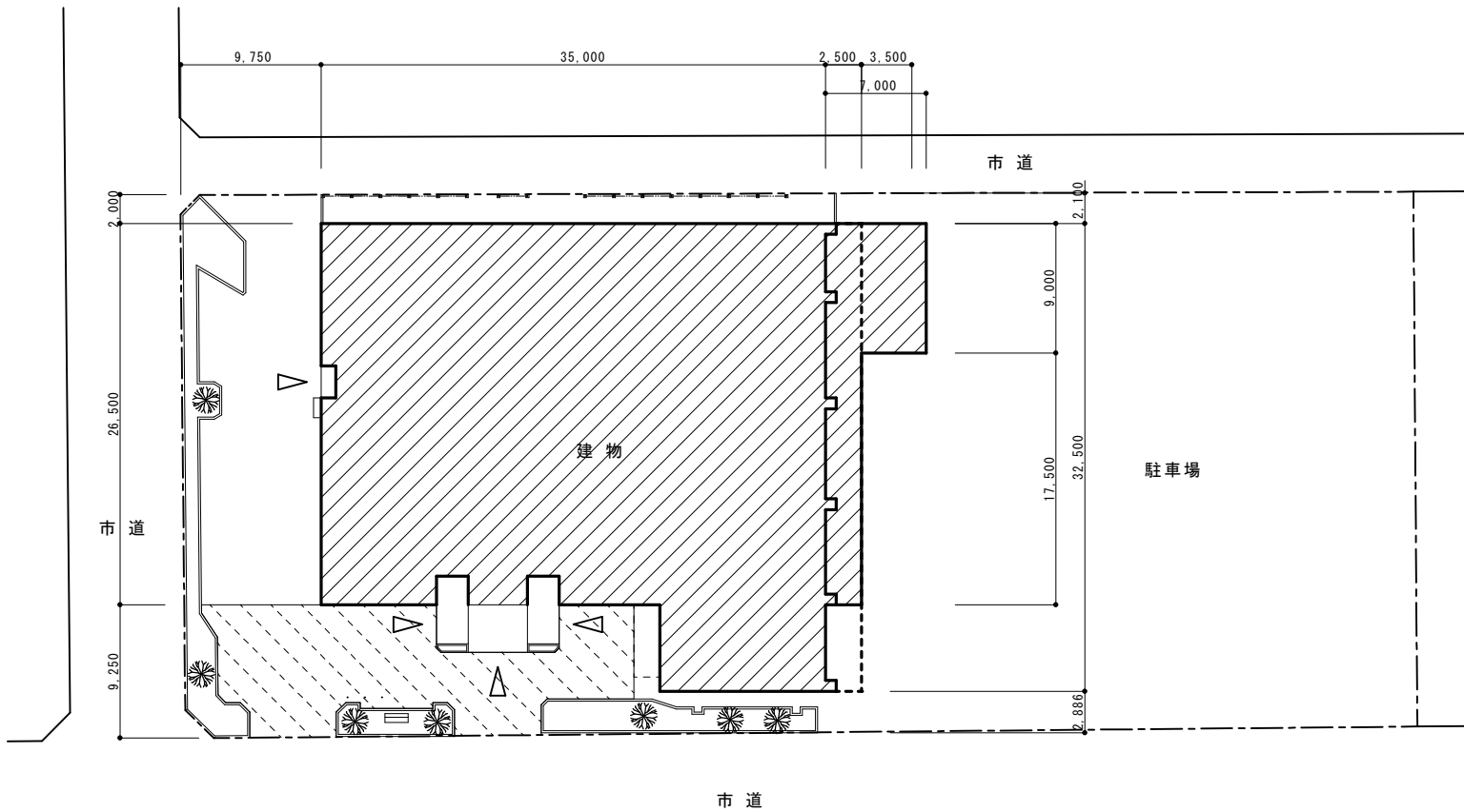
配置図 S=1:1,500
